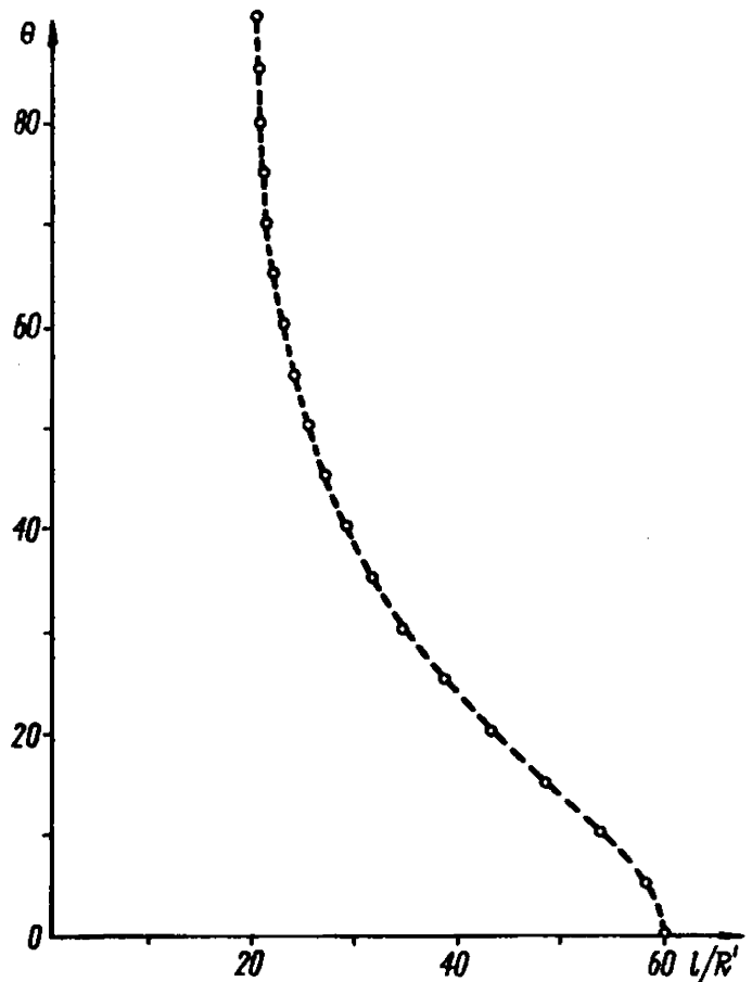
Рис. 10. График изменения величины отношения следа сместителя \sqrt{R'} к его максимальной амплитуде R' от угла \Theta между линией простирания и длиной сместителя
