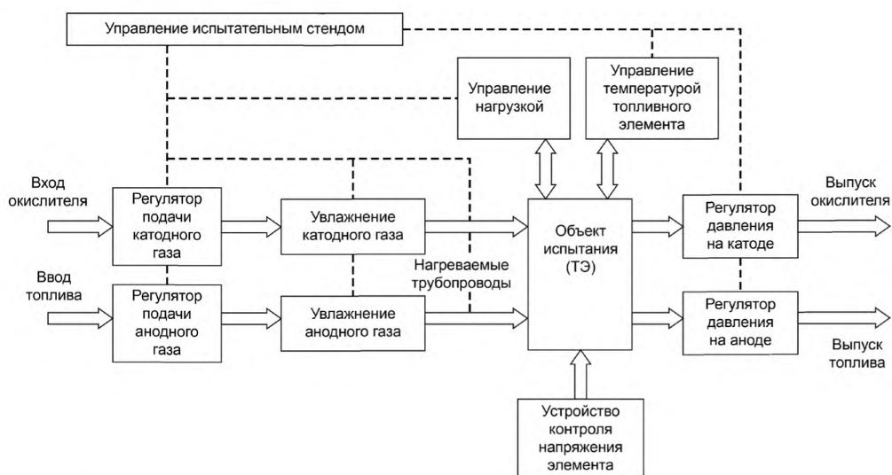
Рисунок 1 — Принципиальная схема стенда для испытания единичного элемента
