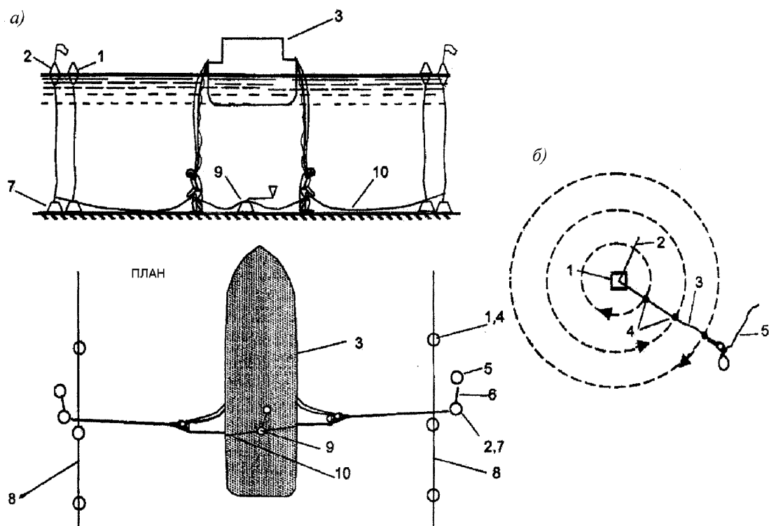
Рисунок Г.1 — Обследование дна акватории водолазами
