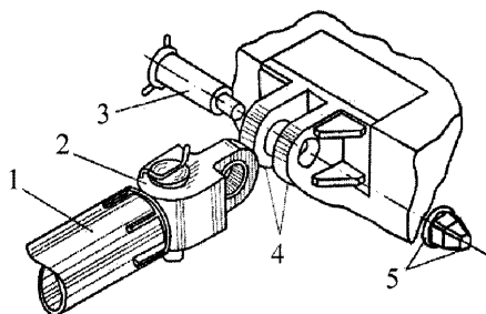
1 – соединительная штанга; 2 – полушарнир штанги; 3 – соединительный палец; 4 – проушины кронштейна понтона; 5 – гайка с шайбой
