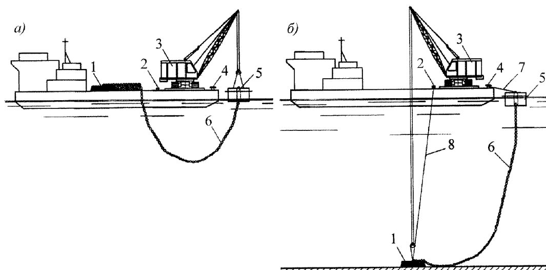
1 – якорь; 2 – лебедка; 3 – грузоподъемное средство; 4 – швартовный кнехт; 5 – рейдовая бочка; 6 – бридель; 7 – швартов; 8 – трос с кольцом
