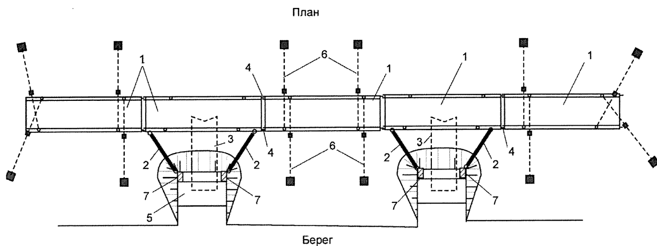
Рисунок А.2 – Типовая схема плавучего причала в виде пирса из крупногабаритных цельнокорпусных понтонов с двумя соединительными штангами
