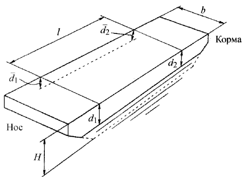
Рисунок 5.1 – Схема измерения осадки, крена и дифферента понтон плавучего сооружения
