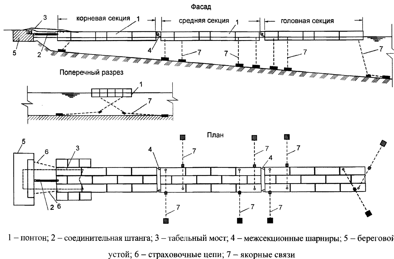
Рисунок А.4 – Типовая схема плавучего причала в виде пирса из малогабаритных понтонов с одной штангой
