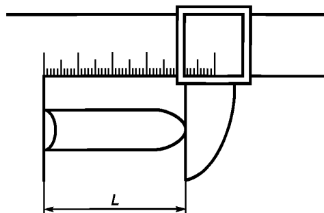
Рисунок 2 — Измерение штангенциркулем длины пеллеты между средней точкой выпуклого конца пеллеты и вогнутым поперечным сечением пеллеты
