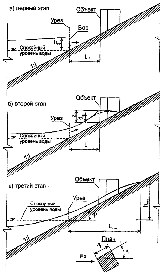
Рисунок 9.1 – Схема воздействия бора на береговой объект
