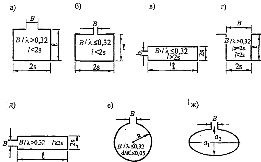
Рисунок Д.3 – Плановые схемы акваторий
