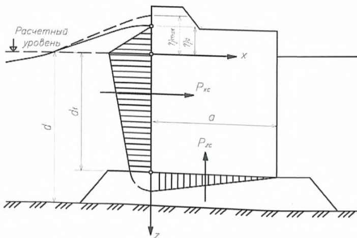
Рисунок 7.2 – Эпюра давления гравитационной волны на вертикальную стенку
