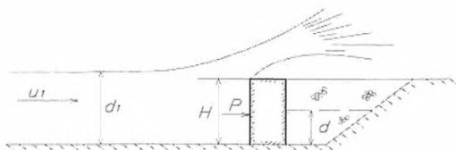
Рисунок 8.3 – Схема взаимодействия бора в фазе удара с причальным сооружением
