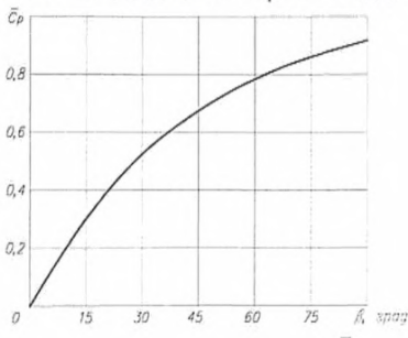
Рисунок 9.6 – Распределение значения коэффициента c_p в зависимости от угла подхода потока к лицевой стороне сооружения прямоугольной формы при L < 5b
