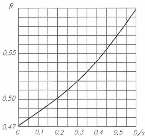
Рисунок 7.6 – График для определения коэффициента R_1
