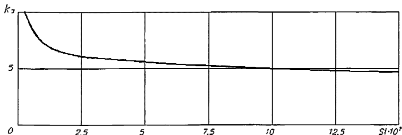
Рисунок 6.7 – График для определения времени затопления
