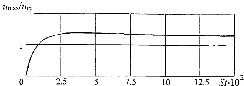
Рисунок 6.4 – График для определения максимальной скорости на урзе при накате волны
