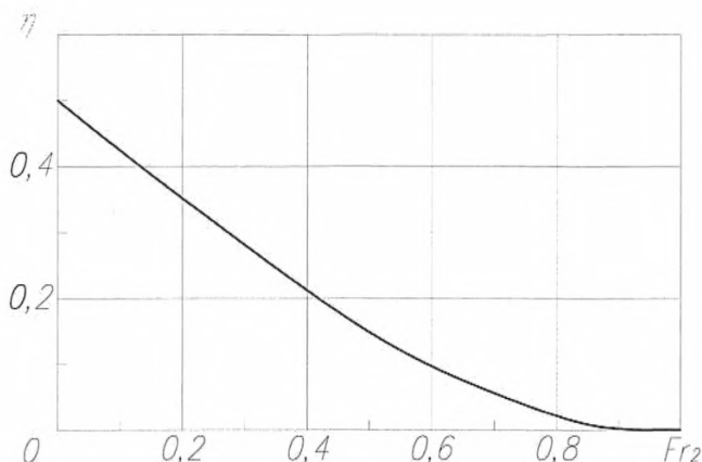
Рисунок 8.11 – График для определения значения \eta
