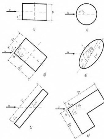
Рисунок 9.4 – Основные типы контуров плохо проницаемых береговых сооружений
