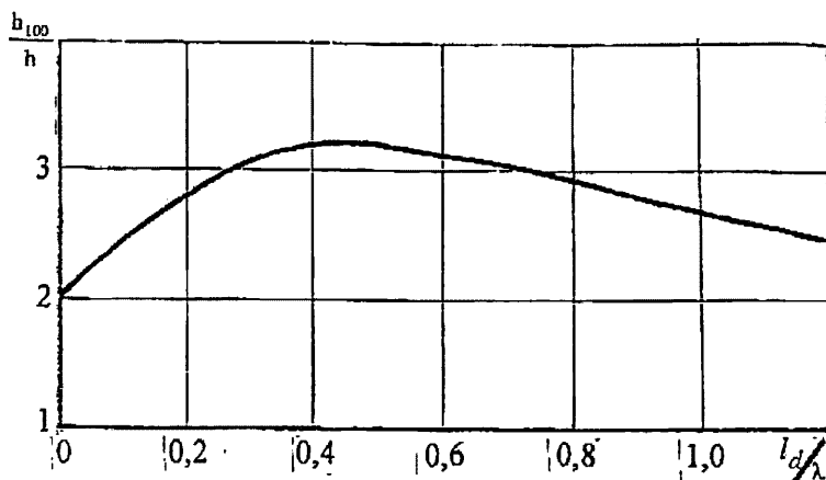
Рисунок Г.1 – График для определения вертикального заплеска
