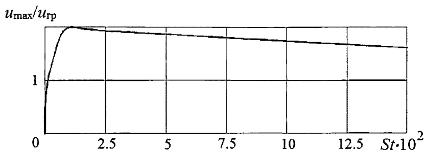
Рисунок 6.5 – График для определения максимальной скорости на урзе при откате волны
