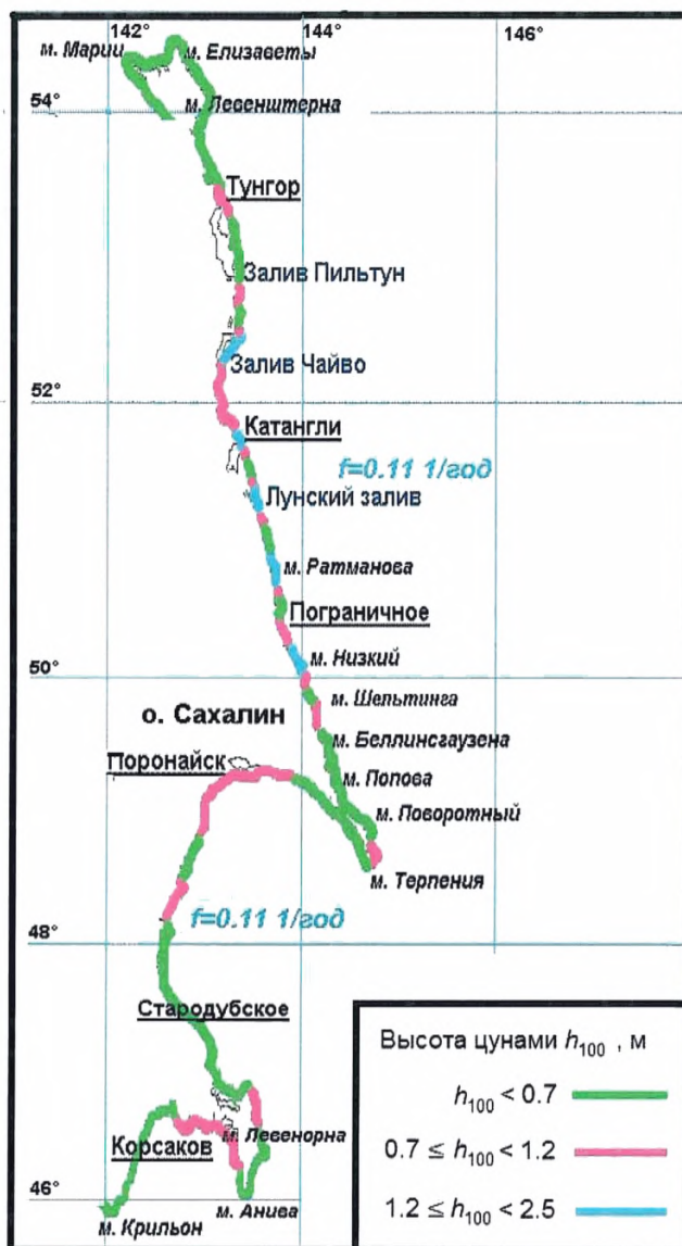
Рисунок А.7 – Карта цунамиопасности восточного побережья о-ва Сахалин
