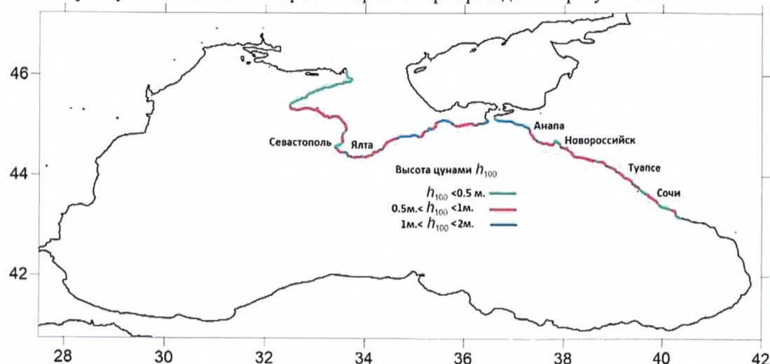
Рисунок А.9 – Карта цунамиопасности побережья Черного моря
