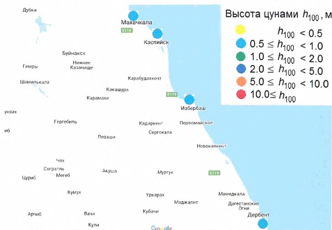
Рисунок А.8 – Карта цунамиопасности побережья Каспийского моря
