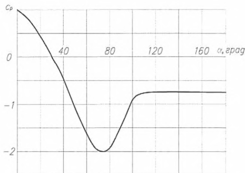
Рисунок 9.9 – Распределение значений c_p по контуру окружности
