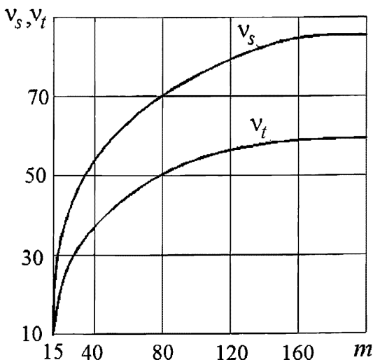
Рисунок 6.8 – Зависимость отношения v_s, v_t от уклона берега
