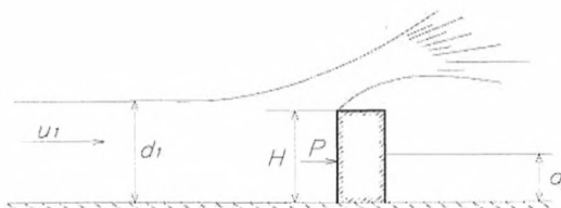
Рисунок 8.2 – Схема взаимодействия бора в фазе удара с ограждающим сооружением
