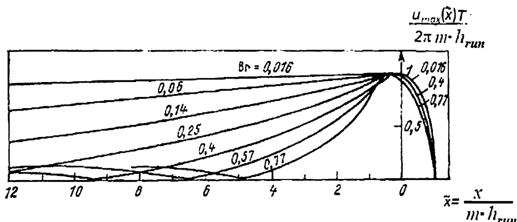
Рисунок 6.2 – Зависимость максимальной безразмерной скорости потока при цунами от безразмерной координаты \bar{x}
