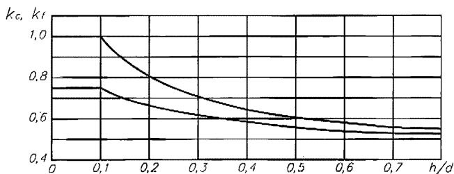
Рисунок 7.1 – Графики значений коэффициентов k_c , k_t
