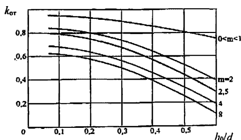
Рисунок Д.1 – График для определения коэффициента отражения k_{от} в зависимости от относительной высоты волны h_0/d и заложения откоса m = \text{ctg} \varphi
