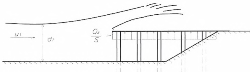
Рисунок 8.12 – Схема взаимодействия бора со сквозным сооружением
