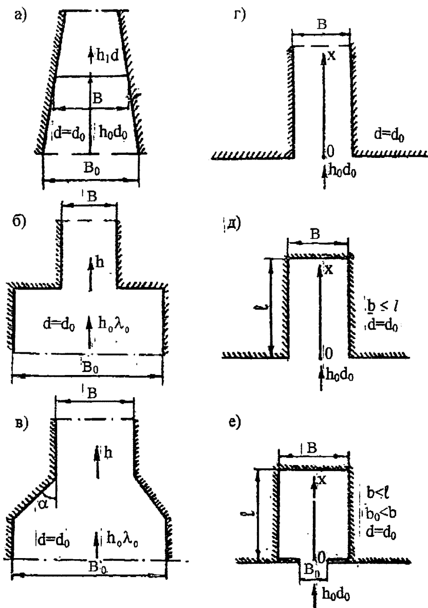
Рисунок Д.2 – К определению высоты волны при изменении геометрических размеров акваторий
