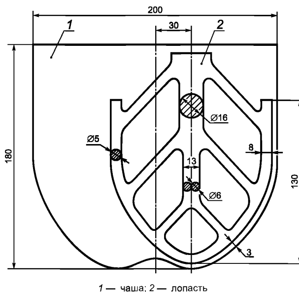
1 — чаша; 2 — лопасть
