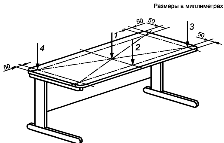
1, 2, 3, 4 — точки приложения нагрузок
