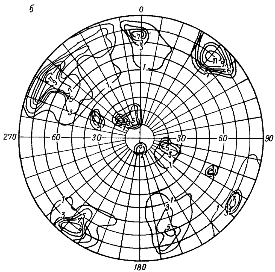
Рис. 29. Круговые диаграммы трещиноватости: a — в полюсах трещин; б — в изолиниях плотности полюсов
