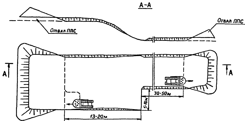
Рис. 4.18. Технология рекультивации непереулаженного прогиба
