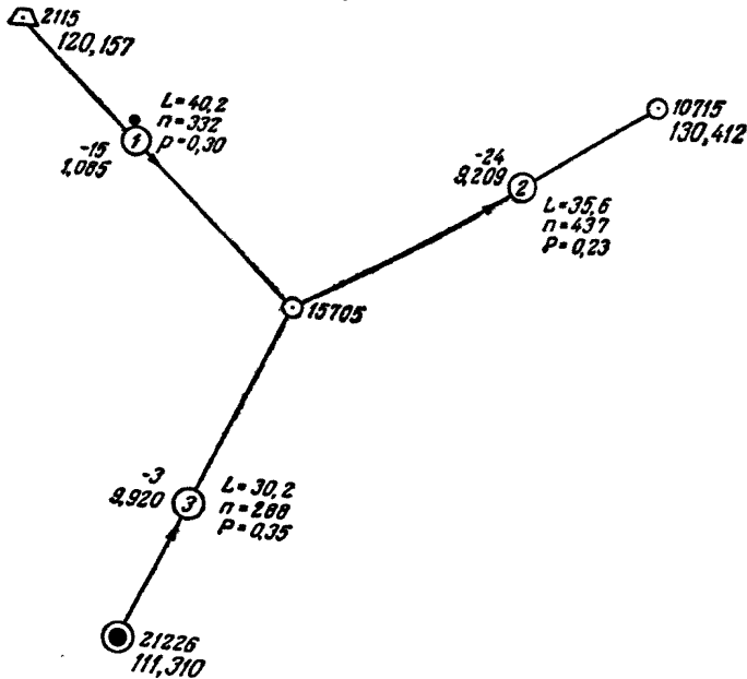
Схема уравнивания линий нивелирования III класса Р-37-67, 68, 79
