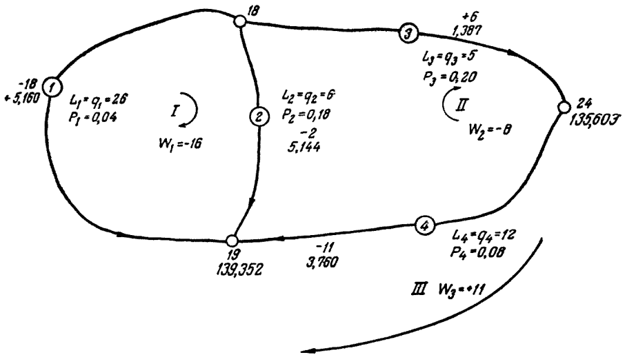
Схема уравнивания линий нивелирования III класса P-37-48
