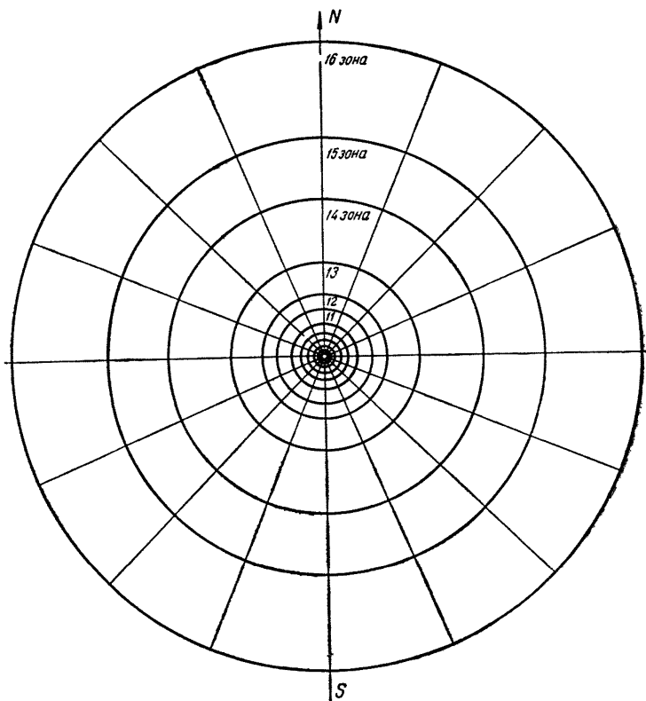
Рис. 2. Палетка для определения средних высот по карте масштаба 1 : 100 000
