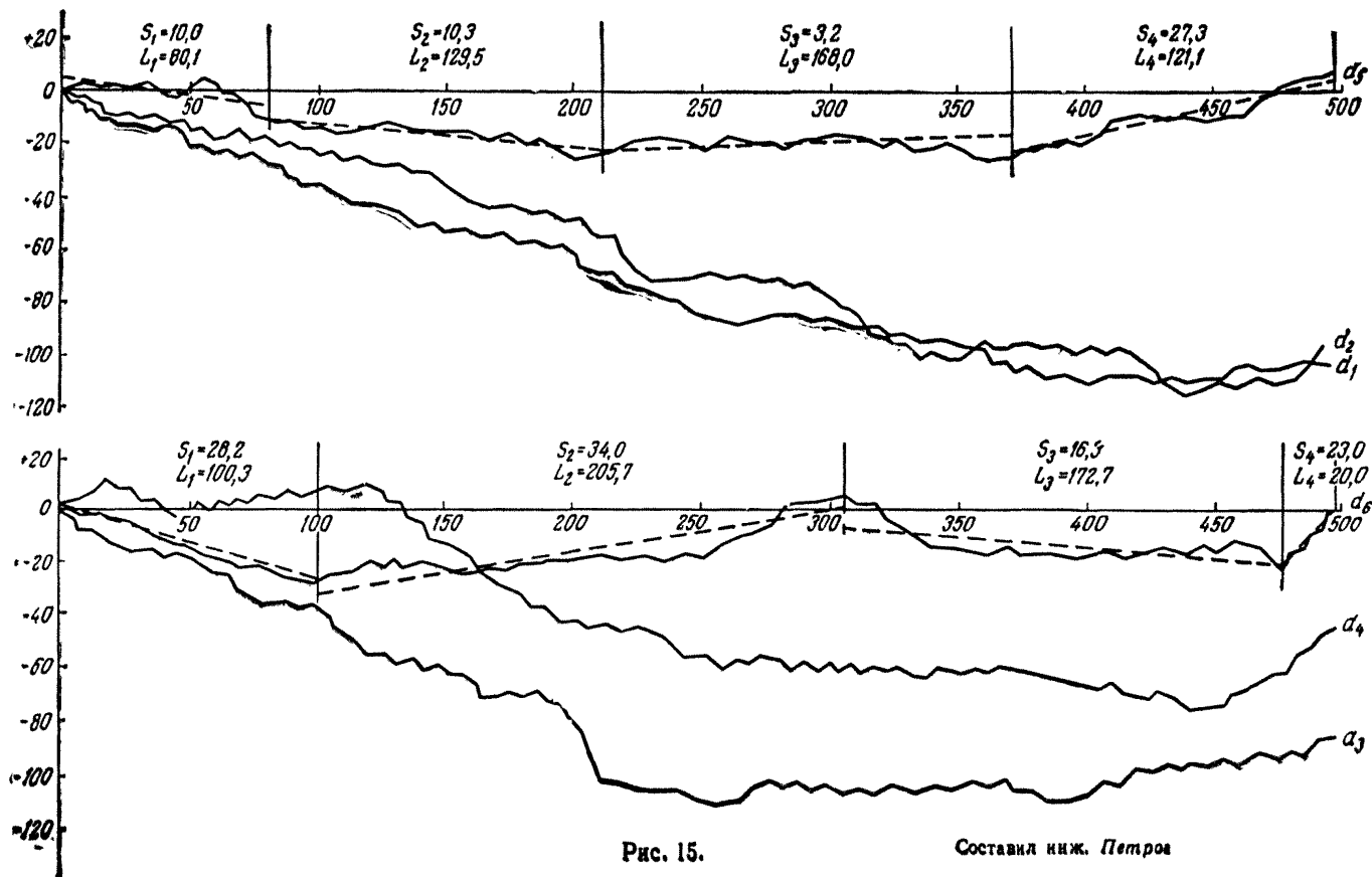
График накопления величин d линия Ивановка — Воробьевка
