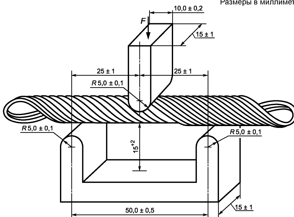
Рисунок 14 — Расположение подставки
