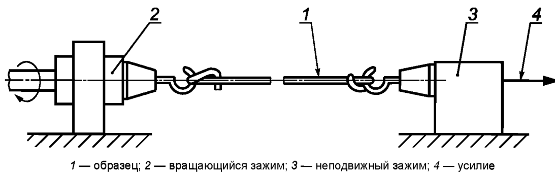
Рисунок 6 — Устройство для испытания на отслаивание
