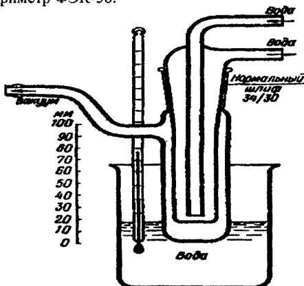
Рис. 10. Прибор для микросублимации.
