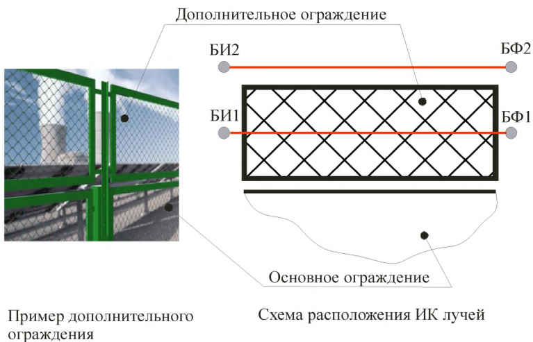
Рисунок 5.15. Схема блокировки верхнего дополнительного ограждения
