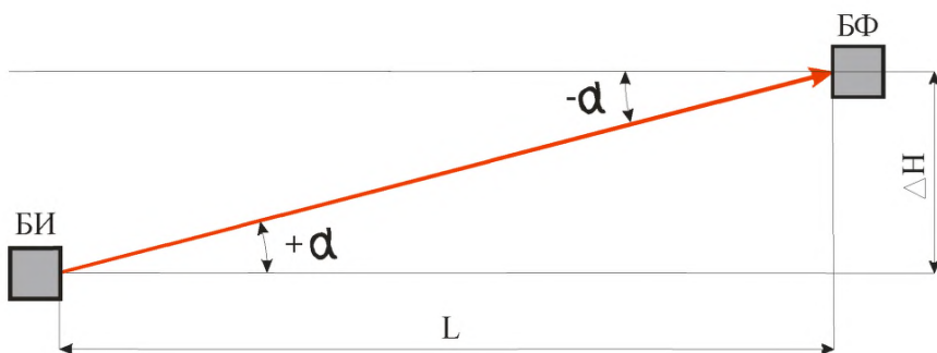
Рисунок 5.3. Схема, поясняющая методику расчета перепада высот установки блоков извещателя
