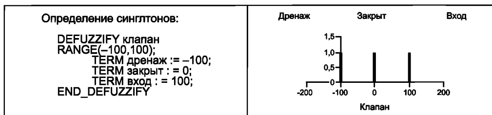
Рисунок 6 — Примеры термов синглтонов
