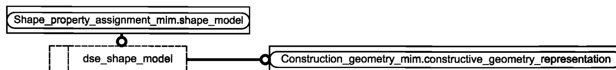
Рисунок D.2 — Представление IMM на уровне объектов в формате EXPRESS-G
