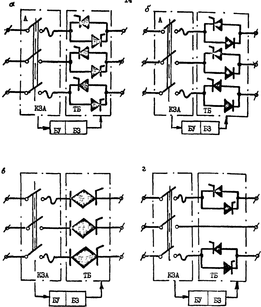
Рис. I. Примеры схем коммутационных аппаратов на силовых приборах:
