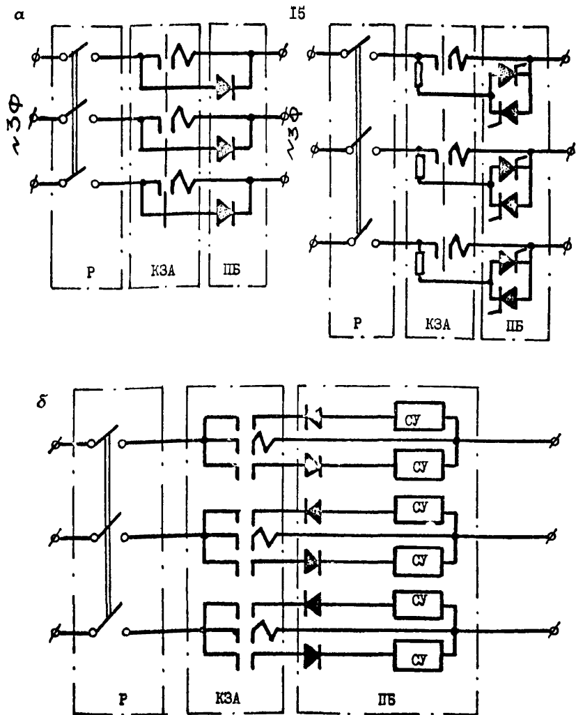
Рис.2. Примеры схем бездуговых коммутационных аппаратов: Р - разъединитель; КЗА - контактный щетчатый аппарат; ПБ - полупроводниковый блок; СУ - синхронное устройство; а - встречное включение вентилялей; б - встречно-параллельное включение тиристоров
