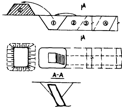
Рис. 3.13. Схема блочной обработки месторождения: 1, 2, 3, ..., n - очередность обработки блоков.
