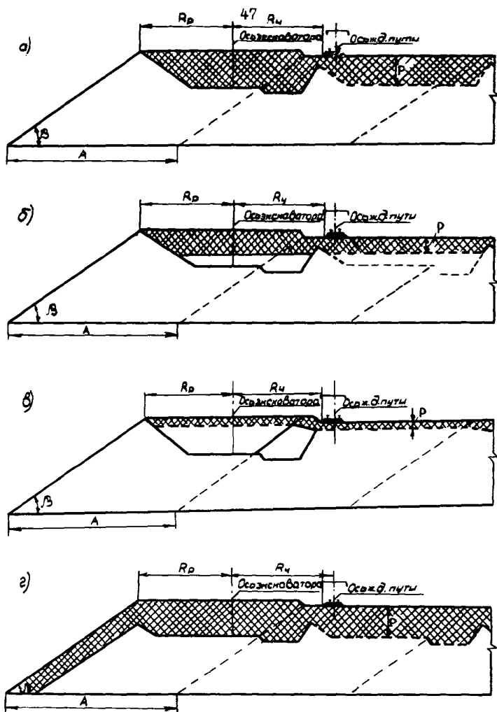
Рис. 3.7. Схемы селективной укатки пород в отвале межплатежи при железнодорожной транспор- те: а - за один проход экскаватора; б - то же, с подступом; в - в комплексе с бульдозером; г - при откатке пород срашно. закладн.
