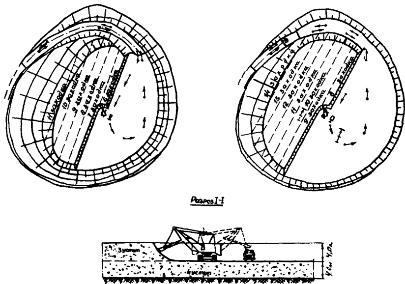
Рис. 4.25. Технология разборки терриконика (выемка породы на 3-ем уступе - прусе, слое).
