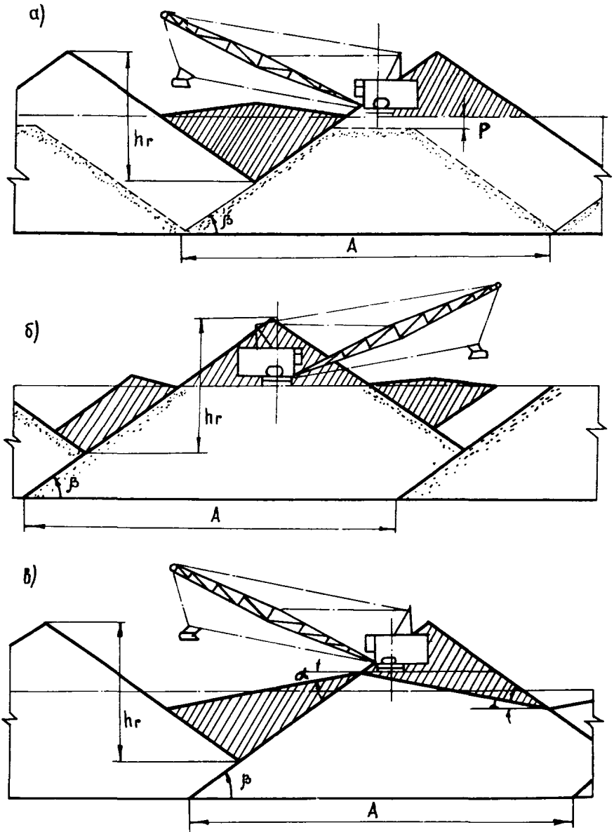
Рис. 3.20. Технологические схемы сплошной планировки отвалов с использованием драглайнов и размещении породы в межгребневом пространстве: а - с одной стороны; б - с двух сторон; в - с одной стороны при волнообразной поверхности.
