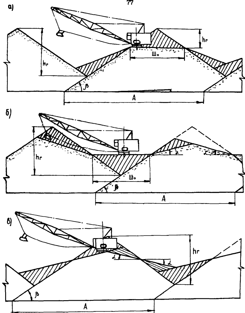
Рис. 3.2I. Технологическая схема частичной планировки отвалов при движении драглайна: а - вдоль границы насыпи и выемки; б - по оси межгребневого пространства; в - по оси гребня.
