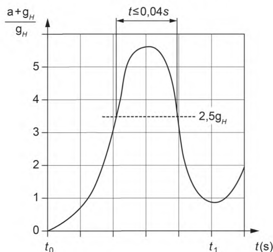
Рисунок А.1 — График торможения
