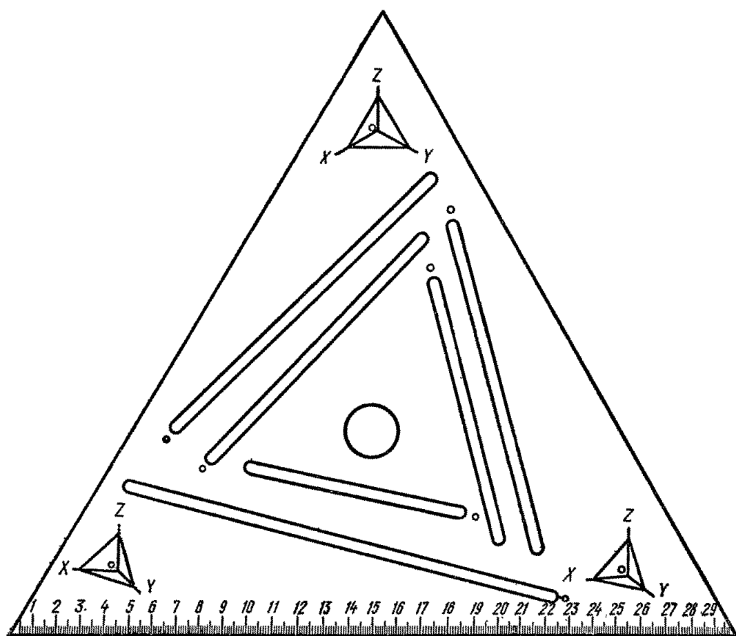
Рис. 12. Штриховальный треугольник
