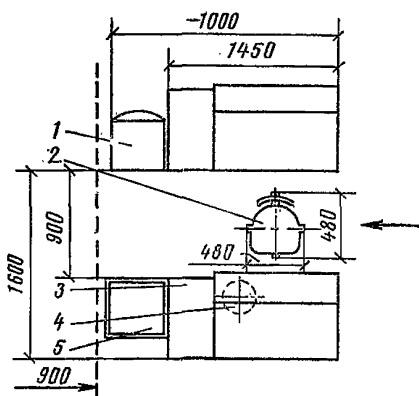
Рис. 12. План рабочего места проектировщика (4-й вариант)
