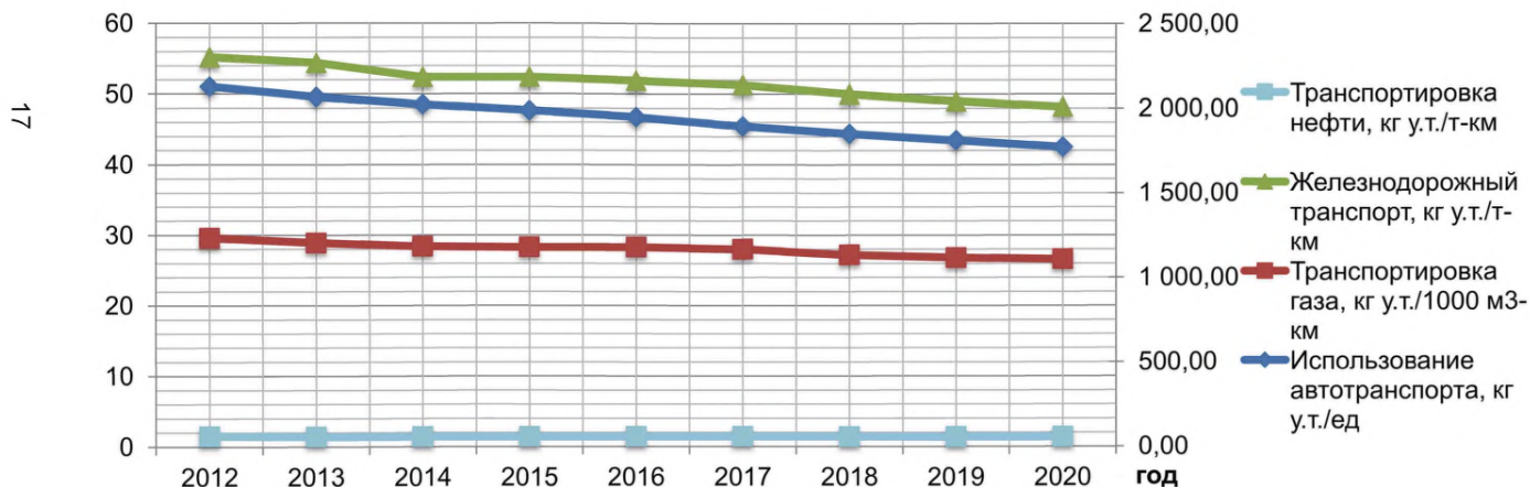
Рисунок 1.2а – Потенциал снижения энергоёмкости отраслей экономики [62]
