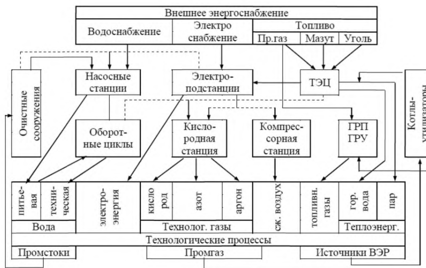
Рисунок 4.1 – Структура энергоснабжения промышленного предприятия
