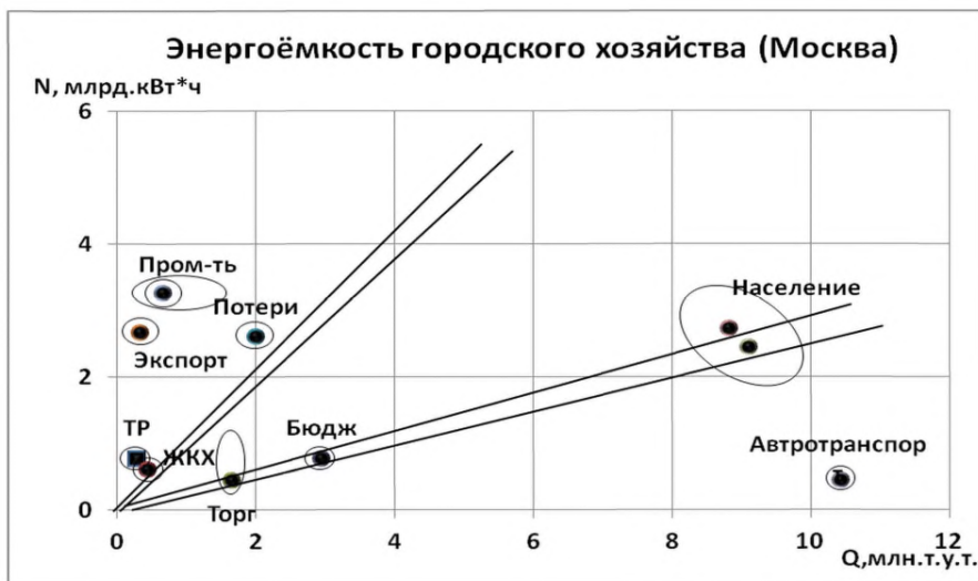
Рисунок 3.3 – Представление ряда секторов городского хозяйства в дипольной диаграмме в координатах – тепло- (топливо) ёмкость и электроёмкость
