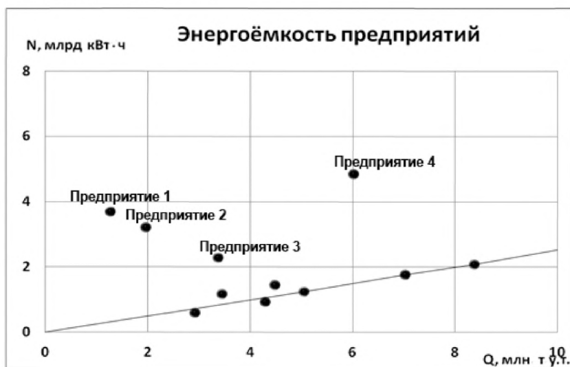
Рисунок 3.2 – Представление отдельных предприятий в дипольной диаграмме энергоёмкости в координатах – тепло- (топливо) ёмкость и электроёмкость
