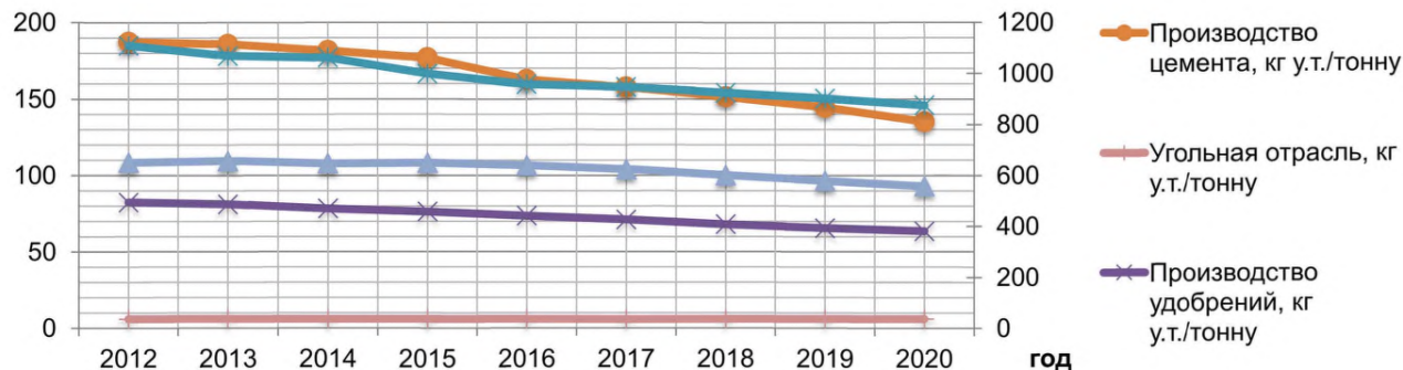
Рисунок 1.26 – Потенциал снижения энергоёмкости отраслей экономики [62]
