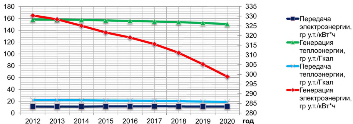
Рисунок 1.2д – Потенциал снижения энергоёмкости отраслей экономики [62]
