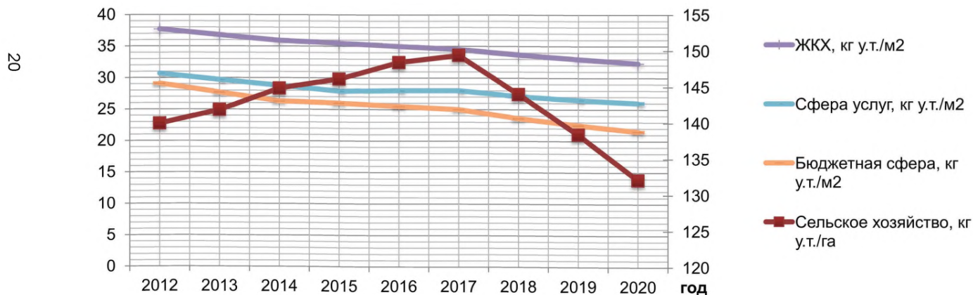
Рисунок 1.2г – Потенциал снижения энергоёмкости отраслей экономики [62]
