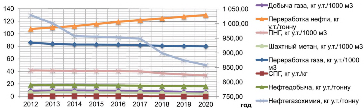
Рисунок 1.2в – Потенциал снижения энергоёмкости отраслей экономики [62]
