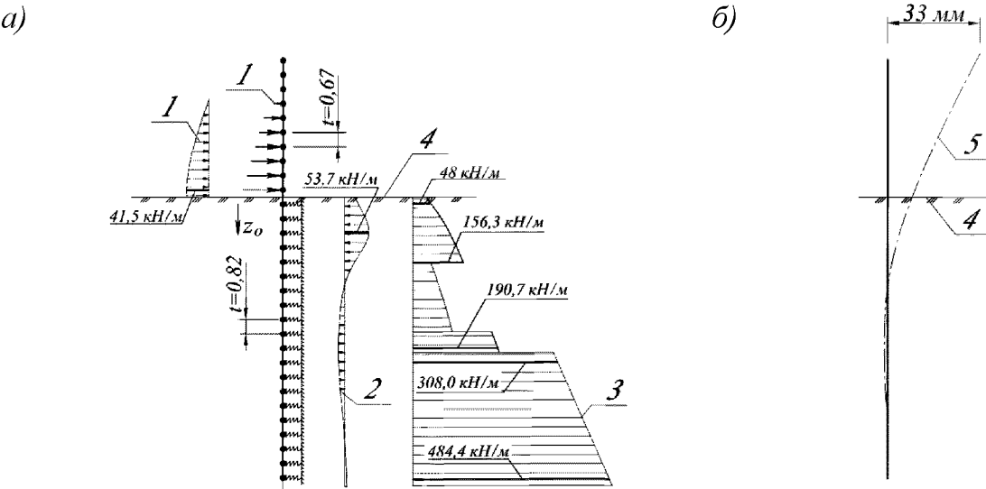
а – расчётная схема и результаты расчёта на первом шаге; б – изогнутая ось ШТС; 1 – эпюра активного давления и узловые силы F_{ai} в надземной части подпорной стенки; 2 – контактное давление P_z = C_z y_z \times I \text{ м} ; 3 – погонная нагрузка P_{пред} ; 4 – планировочная поверхность; 5 – изогнутая ось шпунтовой стенки
