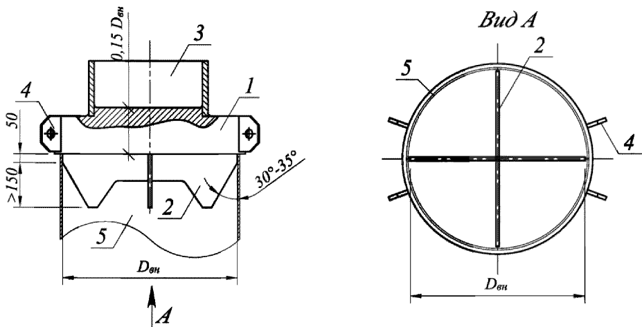
1 – распределительная плита; 2 – фиксирующие уступы; 3 – обойма для размещения амортизатора; 4 – косынки для крепления наголовника к молоту; 5 – трубошпунт
