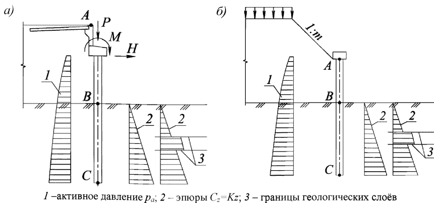
Рисунок В7 – Схемы приложения нагрузок к надземной части устоя (а) и подпорной стенки шпунтового типа (б)
