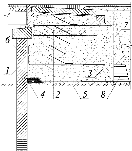
Рисунок 5 – Способ уменьшения горизонтального давления грунта на конструкции ШТС при помощи армогрунтовой системы
