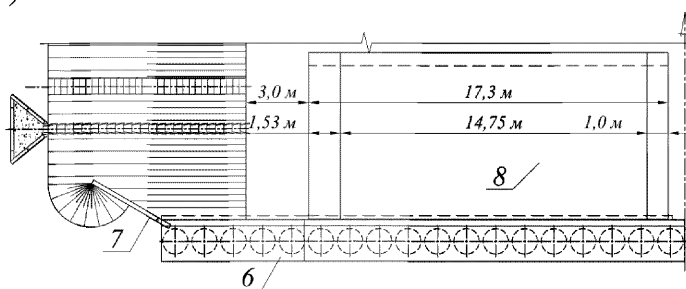
а – фасад опоры ОК1; б – план опоры ОК1
