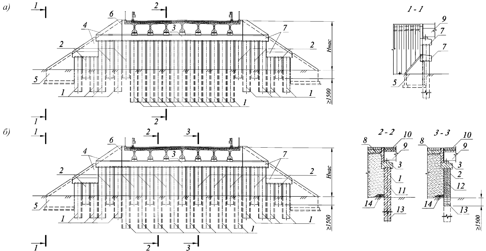
а – устой с непрерывными фундаментными частями; б – устой с прерывистыми фундаментными частями; 1 – несущие (заглубленные) ШТС; 2 – незаглубленные элементы ШТС; 3 – оголовок устоя; 4 – железобетонная стенка; 5 – открылок; 6 – деформационный шов; 7 – железобетонная насадка; 8 – переходная плита; 9 – пролётное строение; 10 – дорожная одежда; 11 – заполнение железобетоном; 12 – заполнение песчано-цементной смесью; 13 – грунтовое ядро; 14 – дренаж
