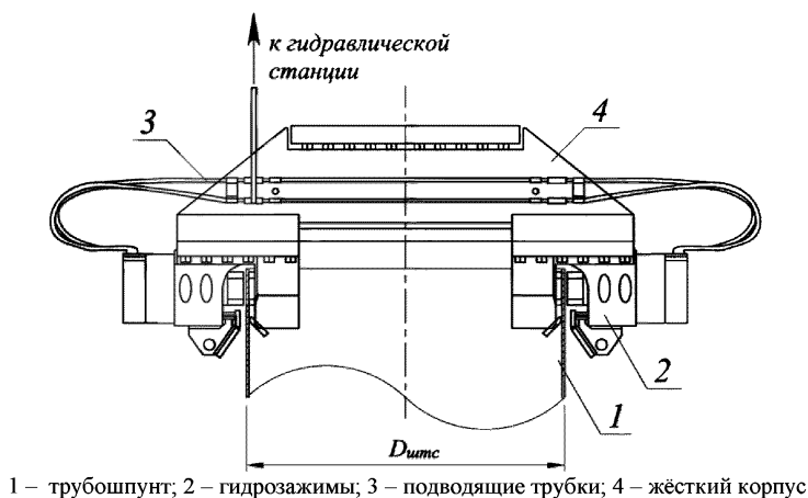
Рисунок 16 – Гидравлический наголовник для вибропогружателя
