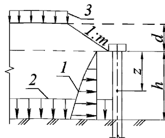
Рисунок В2 – Схема приложения нагрузок к дорожной подпорной стенке из ШТС
