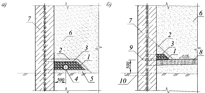
1 – разнофракционный щебень; 2 – гравелистый песок; 3 – геотекстиль; 4 – коллектор (перфорированная труба диаметром 200÷300 мм); 5 – основание из дренирующего грунта; 6 – насыпь (засыпка за устоем); 7 – подпорная стенка (устой моста); 8 – жирная глина; 9 – дренажное отверстие; 10 – железобетонный лоток
