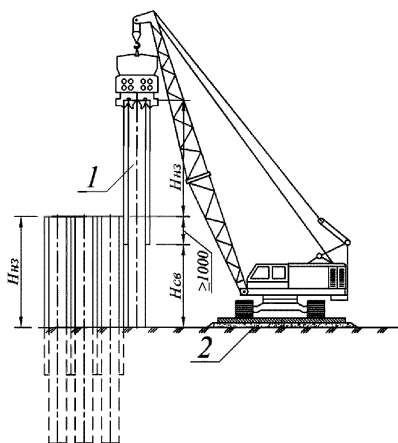
1 – трубошпунт; 2 – планировочная поверхность земли; H_{нз} – высота надземной части сваи, H_{св} – высота свободной от замков части погружаемой сваи
