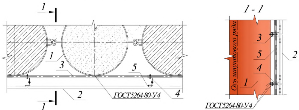
1 – трубошпунт; 2 – облицовка из композитных алюминиевых панелей; 3 – профилированная труба; 4 – кронштейн несущей системы; 5 – направляющая несущей системы
