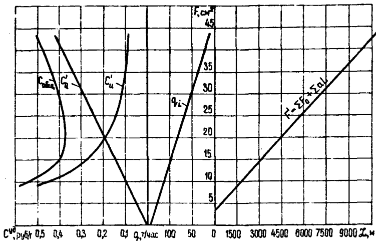
Рис. 2.5. Графики зависимостей: затупления реза от пути резания (трения) \Sigma F = f(L) ; влияния затупления от производительности струга q = f(\Sigma F) и влияния степени затупления резов на себестоимость угля C = f(\Sigma F)
