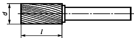
Рисунок 1 — Борфреза типа А
