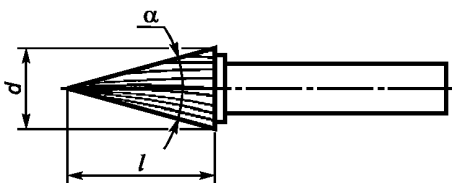
Рисунок 10 — Борфреза типа M
