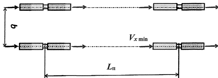
а) Соосная установка струйных вентиляторов
