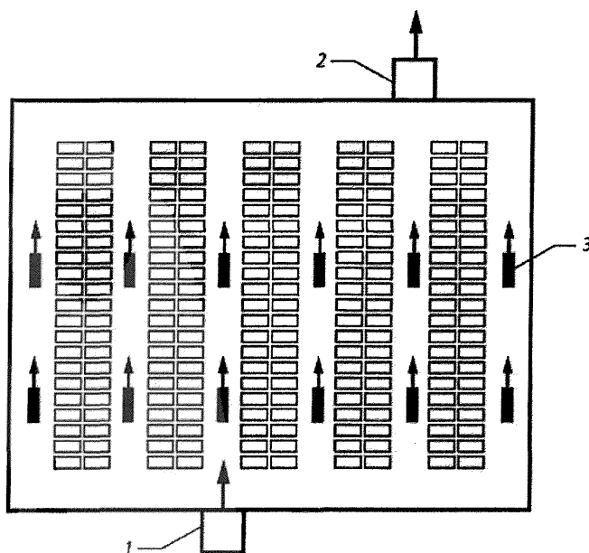
Рисунок 5.3 – Схема работы системы струйной вентиляции в штатном режиме
