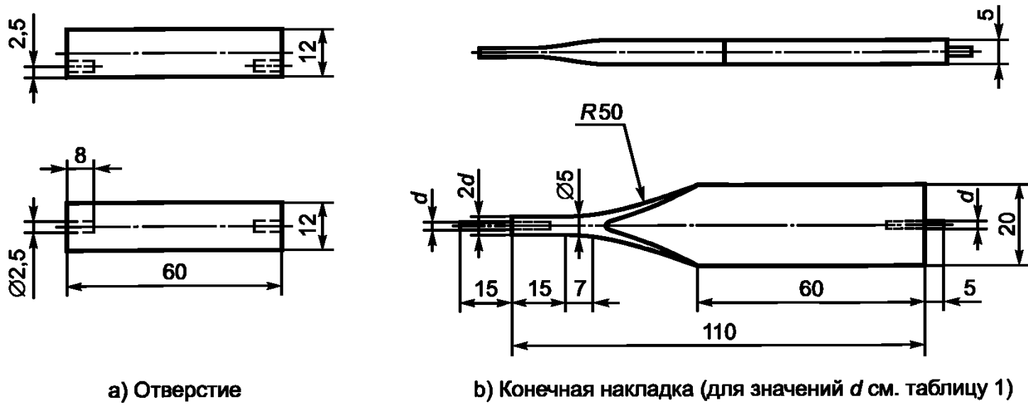
Рисунок 6 — Алюминиевый шаблон
