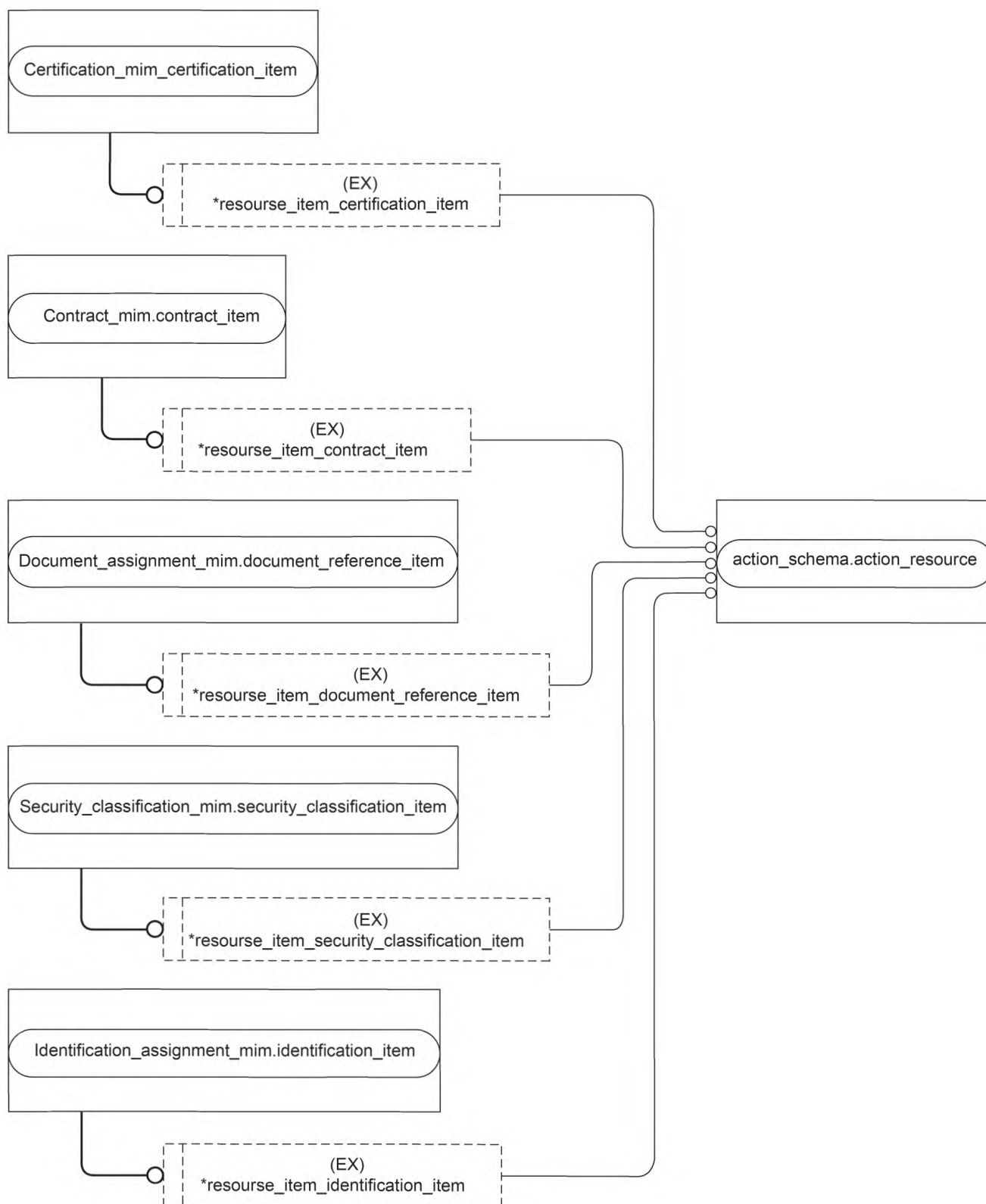
Рисунок D.2 — Представление IMM на уровне объектов в формате EXPRESS-G. Диаграмма 1 из 7
