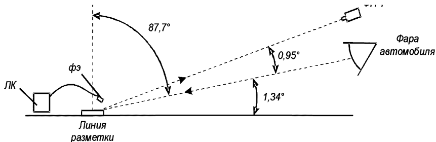
Рисунок 18 – Схема замеров яркости и освещенности горизонтальной разметки от фара автомобиля фотометром
