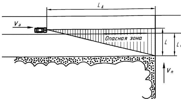
Рисунок 7 – Расчетная схема для определения расстояния боковой видимости
