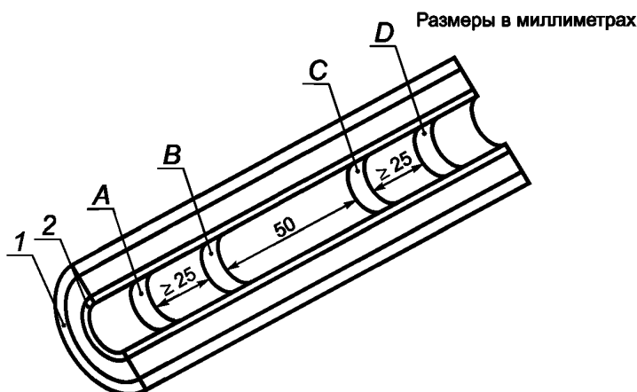
1 — экран по изоляции; 2 — экран по жиле; A, D — электроды тока; B, C — электроды напряжения
