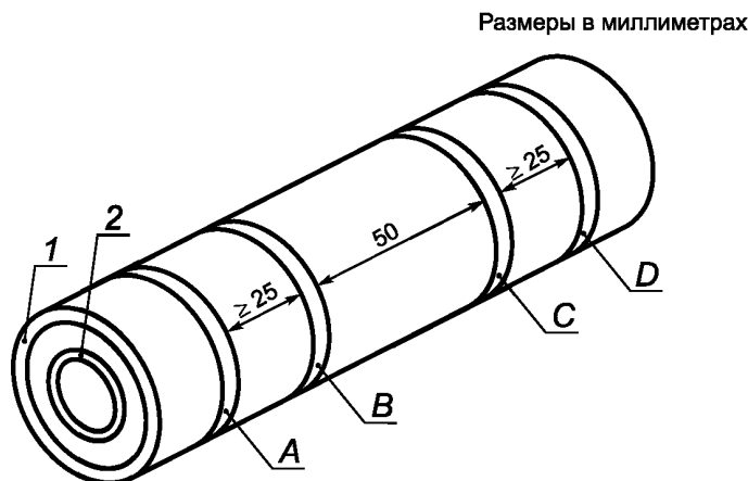
1 — экран по изоляции; 2 — экран по жиле; A, D — электроды тока; B, C — электроды напряжения
