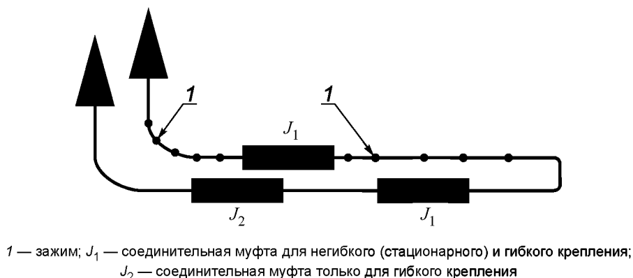
Рисунок 1 — Пример испытательной установки для проведения предквалификационного испытания
