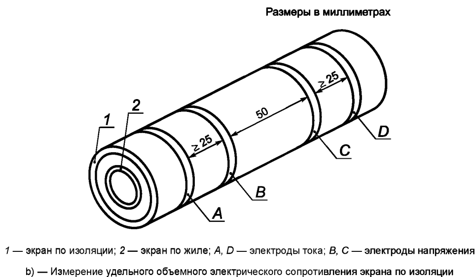
Рисунок D.1 — Подготовка образцов для измерения удельного объемного электрического сопротивления экранов по жиле и по изоляции
