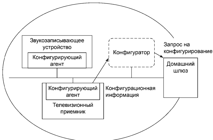
Рисунок 2 — Информационные и конфигурационные требования модели конфигуратора
