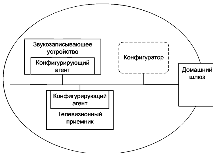
Рисунок 1 — Модель системы конфигуратора
