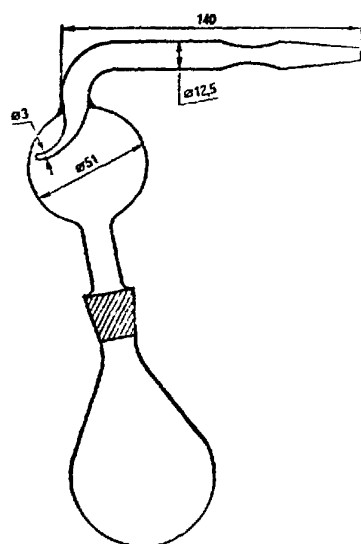
Рис. 19. Каплеуловитель — прибор для ускоренного концентрирования экстракта (размеры в мм).
