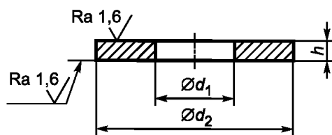
Рисунок 1 — Шайба типа S
