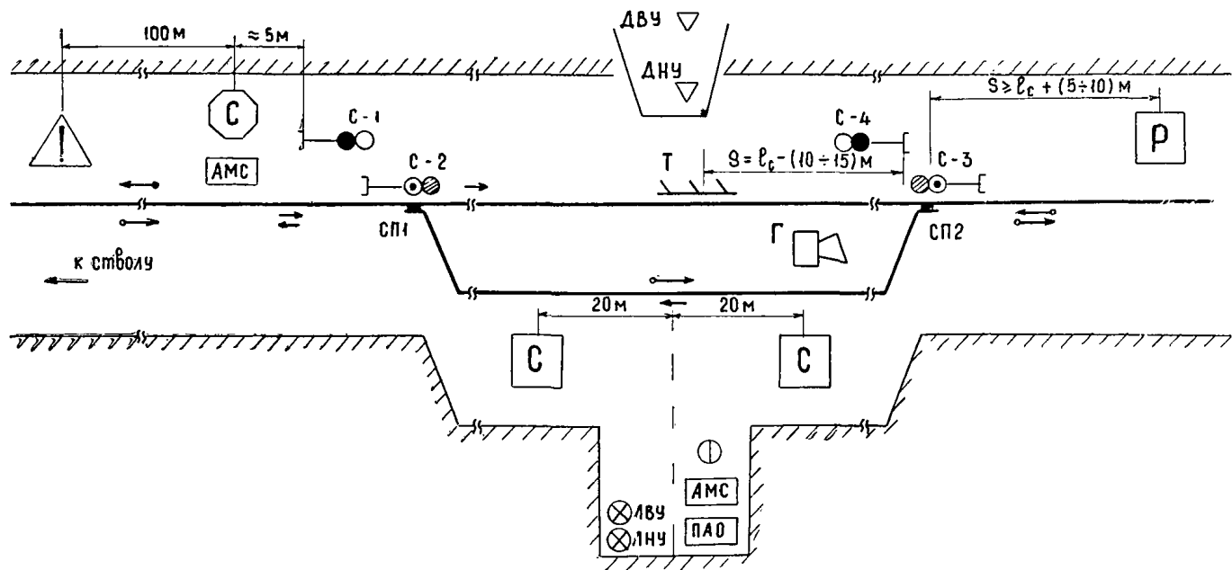
Рис. П.3.1. Схема расстановки средств сигнализации на стационарном погрузочном пункте в однопутевой выработке с обменной разминковкой под погрузкой. l_c — длина состава вагонеток
