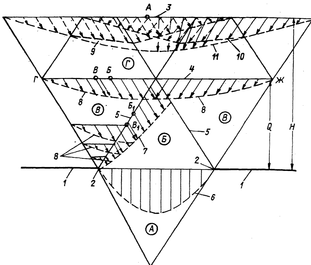
Рис. I.5. Схема перемещений покрывающей толщи на нормальном к напластованию разрезе по простиранию пласта:
