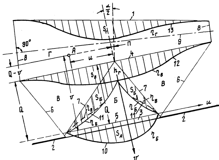
Рис. I.4. Схема перемещений подрабатываемого горного массива на вертикальном разрезе вкrest простирания пласта:
