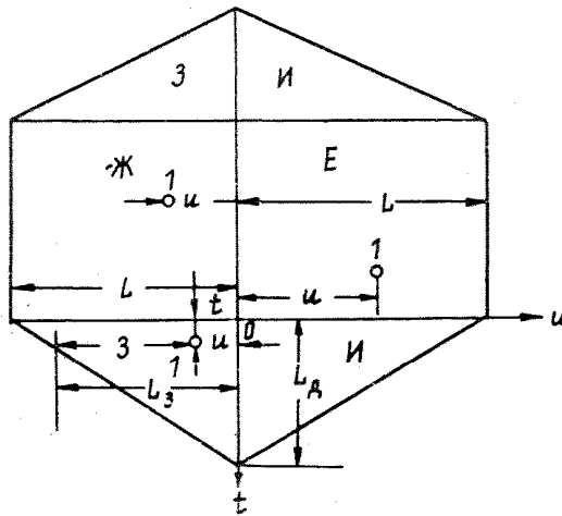
Рис. 1.6. Схема подработанного массива на разрезе по напластованию, поясняющая способ определения относительной координаты точки 1, лежащей на участке 3, или И, или Д:
