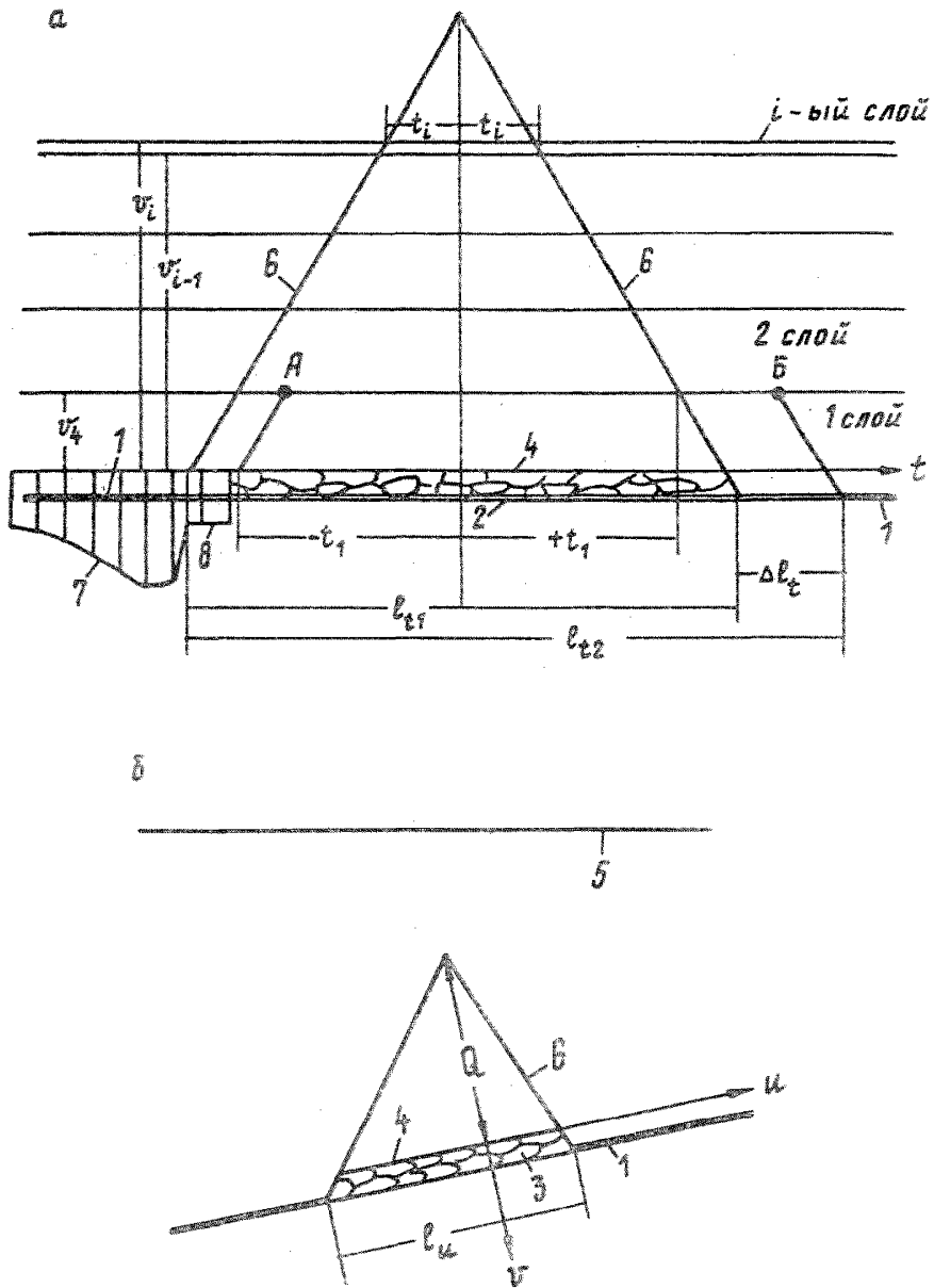
Рис. I.I. Расчетная схема подработанного массива горных пород:
