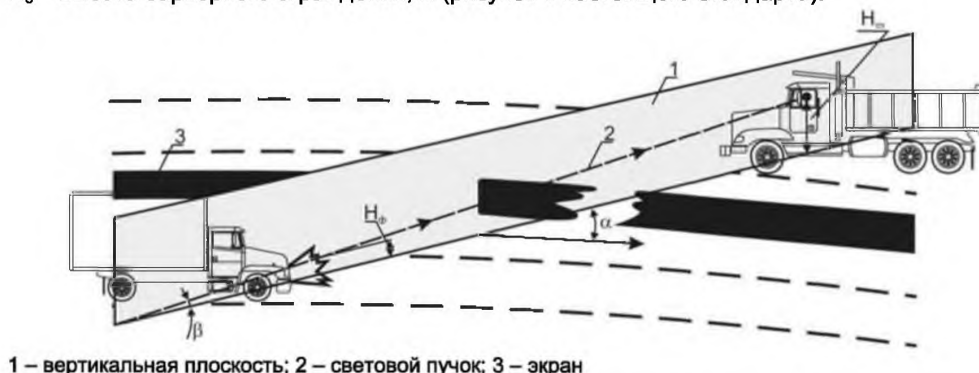
Рисунок А.1 – Схема расположения транспортных средств в вертикальной плоскости
