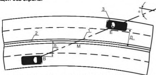
Рисунок А.2 – Схема расположения транспортных средств в плане
