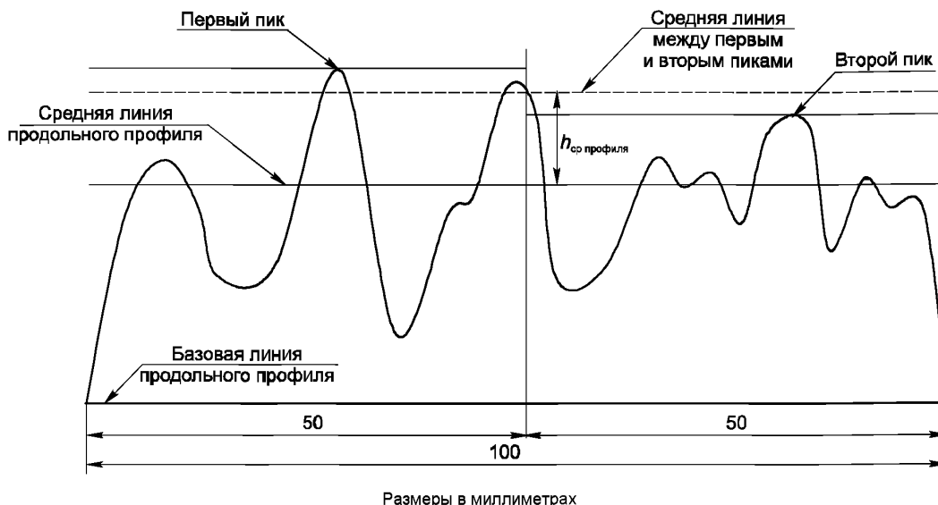
Рисунок 5 — Схема к алгоритму обработки результатов измерений шероховатости дорожного покрытия методом профилирования
