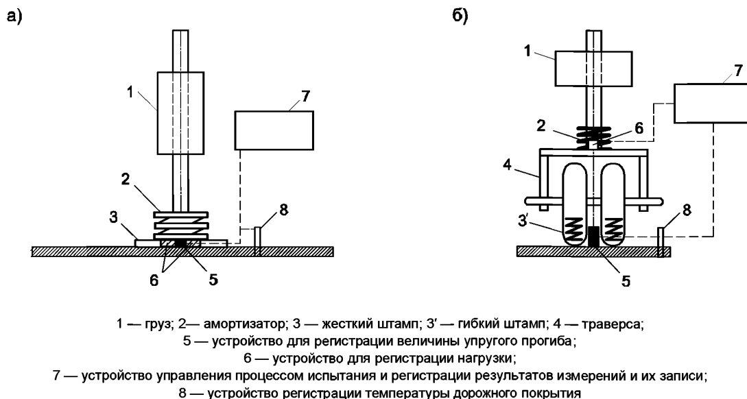
Рисунок 2 — Схема проведения испытаний по определению упругого прогиба динамическим методом:
