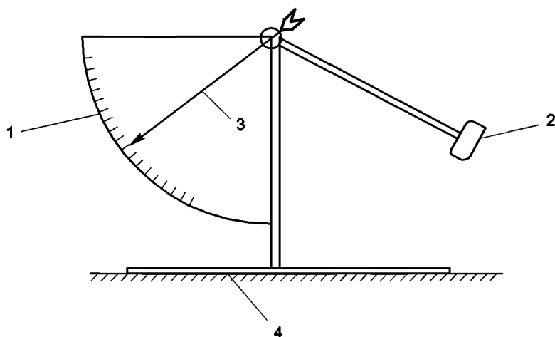
1 — шкала прибора; 2 — маятник; 3 — стрелка; 4 — мокрое покрытие
