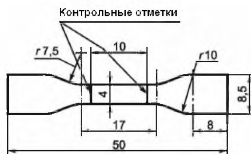
Рисунок 4 – Образец в виде двусторонней лопатки с меньшими размерами
