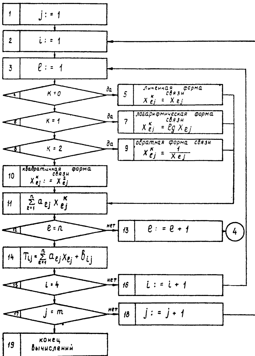
Блок-схема алгоритма расчёта трудоёмкости по процессам и звеньям производства карьера.
