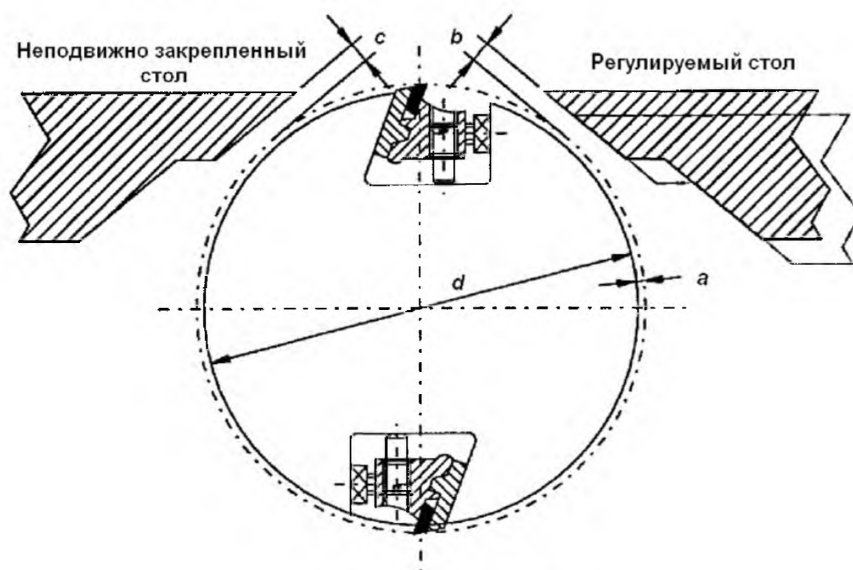
Рисунок 101 – Ножевой блок
