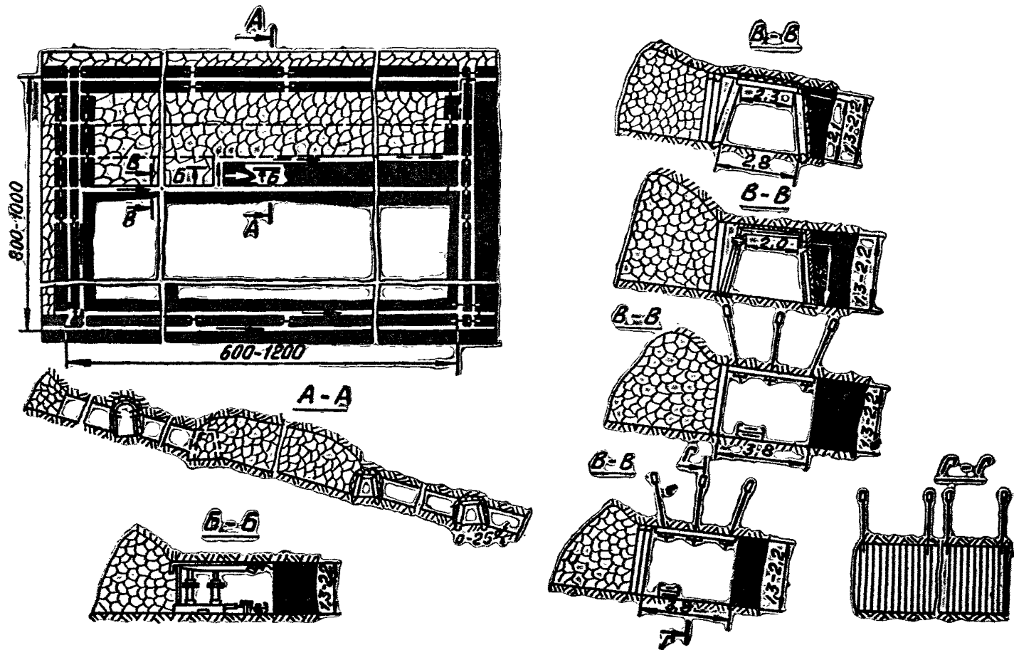
Рис. 3-1. Схема подготовки и отработки выемочных полей с сохранением конвейерного штрека на полное сечение на пластах средней мощности
