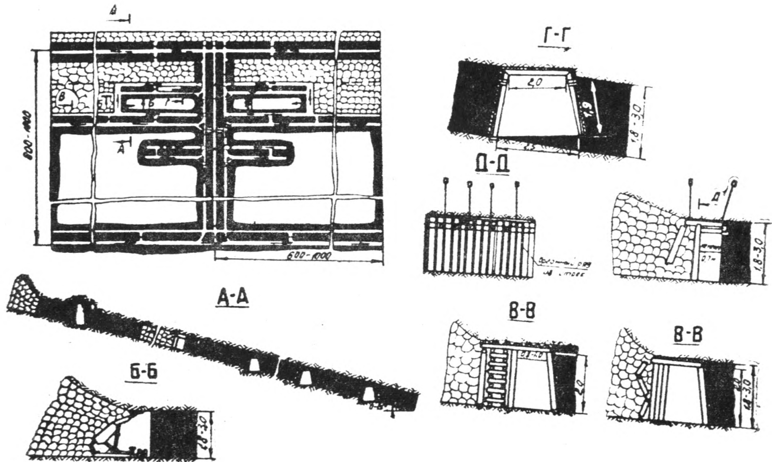
Рис. 3-10. Схема подготовки и отработки выемочных сечений и выемкой подэтажных цеколов:
