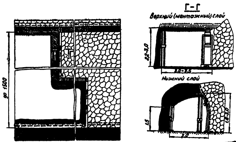
Рис. 3. 9. Схема подготовки и отработки выемочных полей с проходкой вентиляционной (конвейерной) выработки позади очистного забоя при разработке мощных пластов наклонными слоями с применением гибких перекрытий и крепи КТУ
