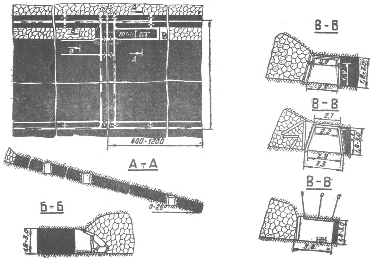
Рис. 2-1. Схема подготовки и отработки двухсторонних бремсберговых (уклонных) полей с проходкой вентиляционных штреков по контакту с обрушенными породами
