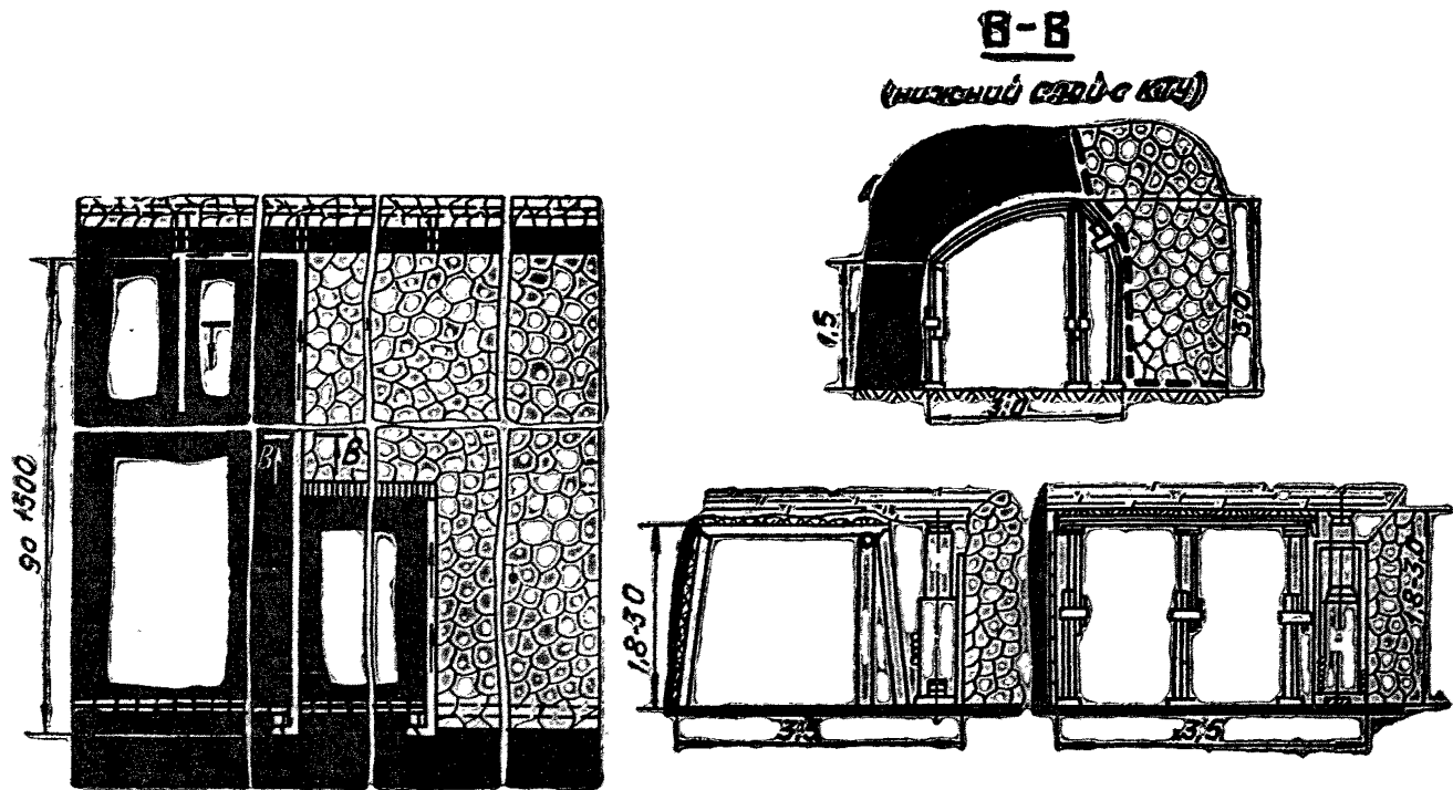
Рис. 3-3. Схема подготовки и отработки выемочных полей с сохранением конвейерной печи у границы с выработанным пространством при разработке мощных пластов наклонными слоями с применением гибких перекрытий и крепи КТВ
