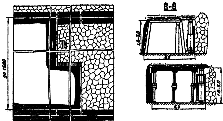
Рис. 3.8. Схема подготовки и отработки выемочных полей с проходкой вентиляционной (конвейерной) выработки одновременно с очистным забоем при разработке пластов средней мощности длинными столбами по падению
