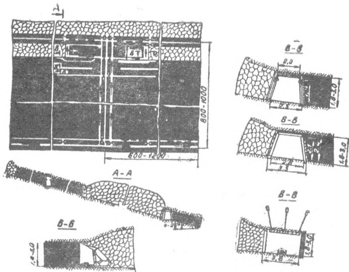
Рис. 2.2. Схема подготовки и отработки двухсторонних бремсберговых (уклонных) полей с проходкой вентиляционных штреков по контакту с обрушенными породами встречными забоями к продвижению верхних лав
