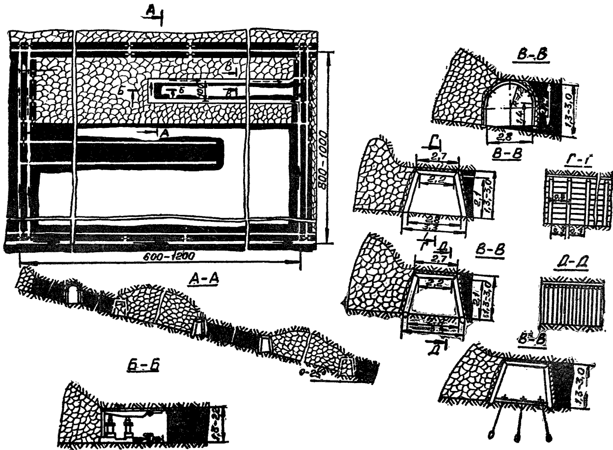
Рис. 24. Схема подготовки и отработки односторонних бремсберговых (уклонных) полей с проходкой оконуривающих выработок промежуточной лавы после отработки выше- и нижележащей лав
