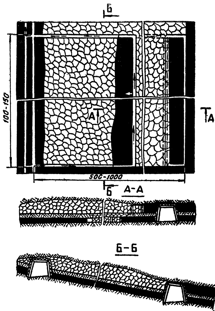
Рис. 3.12. Схема подготовки и отработки весьма сближенных тонких пологих или средней мощности пластов, разделенных породным прослоем, с сохранением оконтуривающих выработок для нижнего слоя
