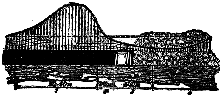
Рис. 1-1. Распределение зон горного давления: 1—зона опорного давления; 2—зона разрушения угля; 3—зона, разгруженная от опорного давления; 4—зона уплотнения обрушенных пород
