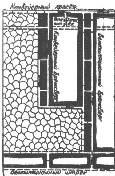
Рис. 3.11. Схема подготовки и отработки выемочных полей с проходкой вентиляционного штрека (бремсберга) по контакту с выработанным пространством и выемкой подэтажных целиков механизированными комплексами
