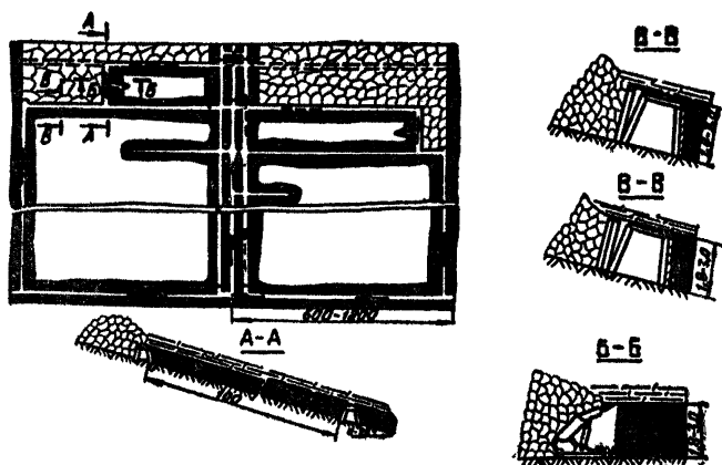
Рис. 3.5. Схема подготовки и отработки бремсберговых (уклонных) полей с сохранением конвейерного штрека и проветриванием его по разрезной печи с основного штрека
