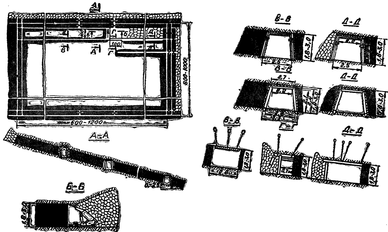
Рис. 2.3. Схема подготовки и обработки односторонних бремсберговых (уклонных) полей с проходкой вентиляционных штреков с отставанием от очистного забоя вышележащей лавы
