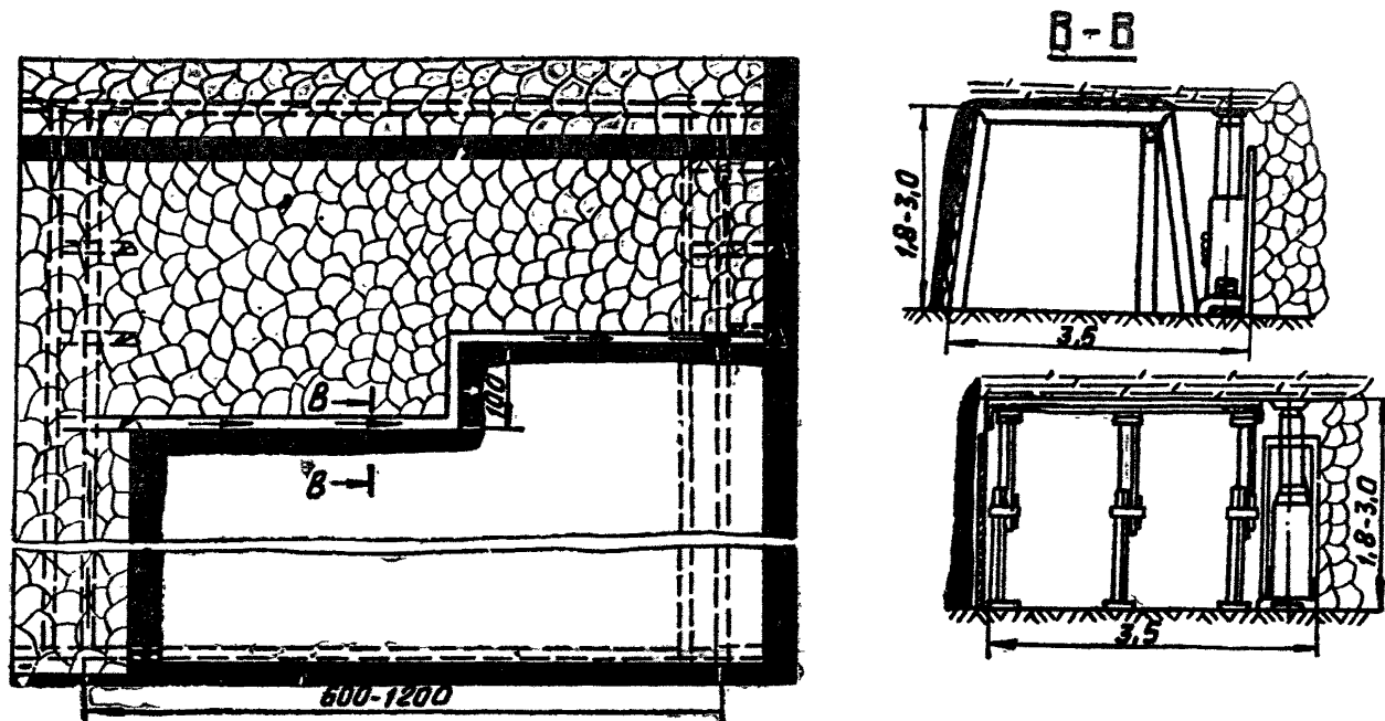
Рис. 3.7. Схема подготовки и отработки выемочных полей с проведением конвейерного штрака позади очистного забоя по контакту с выработанным пространством при разработке мощных пластов
