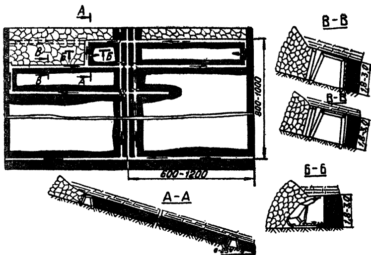
Рис. 3.4. Схема подготовки и отработки бремсберговых (уклонных) полей с сохранением конвейерного штрека и проветриванием его по конвейерному штреку и разрезной печи шихележащей лавы
