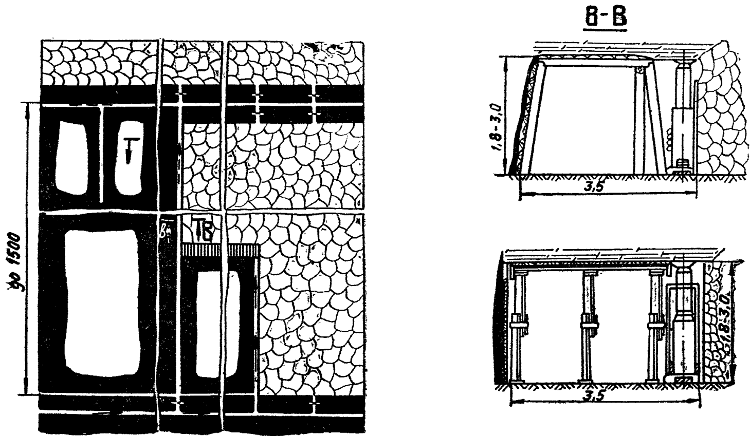
23 Рис. 3-2. Схема подготовки и отработки выемочных полей с сохранением конвейерной печи у границы с выработанным пространством на пластах средней мощности
