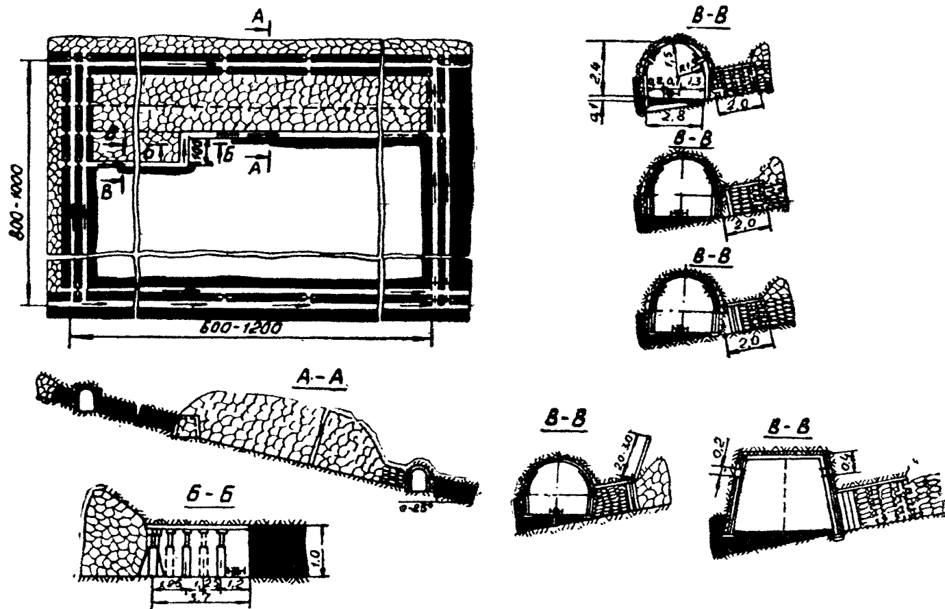
Рис. 36 Схема подготовки и отработки выемочных полей с проведением конвейерного штрека позади очистного забоя по контакту с выработанным пространством при разработке пологих пластов мощностью до 1,5 м
