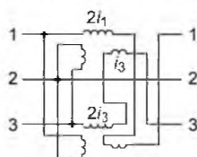
Рисунок 2 – Соединение с перекрестной фазой счетчика вар-часов с двумя измерительными элементами и цепи расщепленного тока в трехфазных трехпроводных цепях
