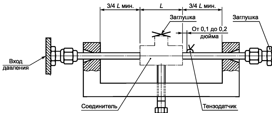
б) Испытательная установка для соединителя типа Т
