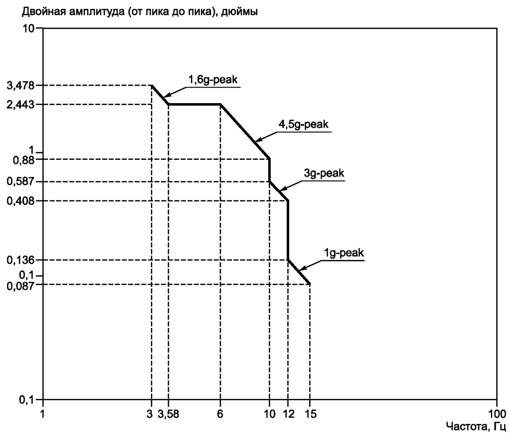
Рисунок 12 — Кривая 3А
