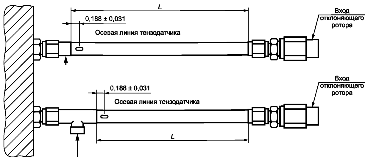
Рисунок 3 — Образец при импульсных испытаниях с кручением
