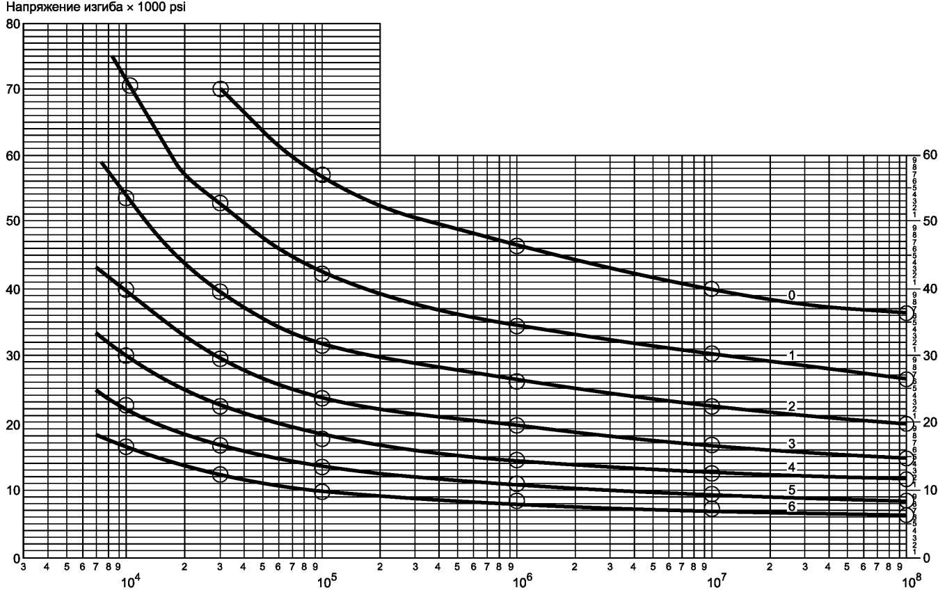
Рисунок 2 — S/N кривая испытания на разрушение при изгибе
