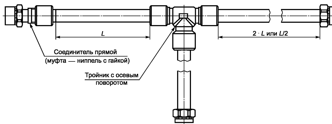
Рисунок 1 — Конфигурация соединения труб для проведения импульсных испытаний
