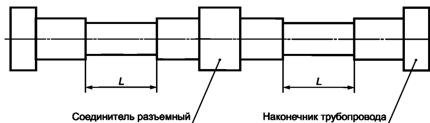
Рисунок 14 — Длины испытываемых образцов для испытаний на коррозионно-усталостные трещины
