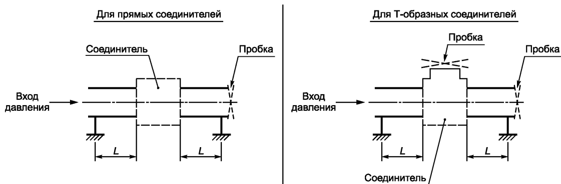
Рисунок 6 — Установка для испытаний на вибрацию
