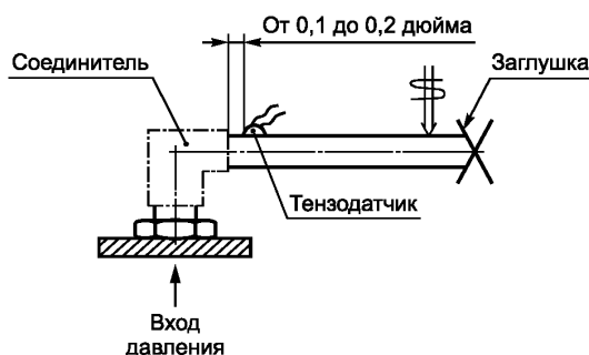
в) Испытательная установка для углового соединителя
