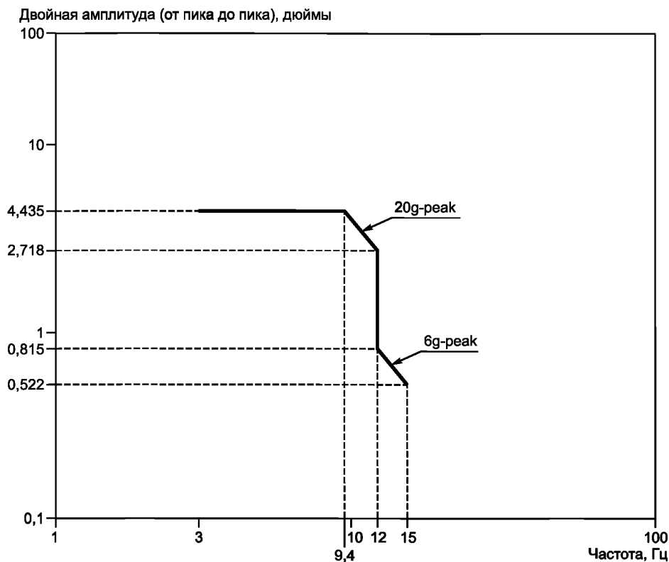
Рисунок 13 — Кривая 5В
