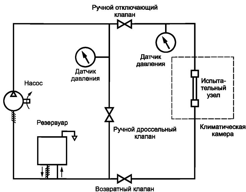
Рисунок 4 — Типовая установка для испытаний на термостойкость
