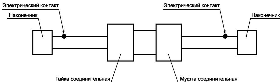
Рисунок 15 — Образец для испытаний на удар молнии. Труба в сборе
