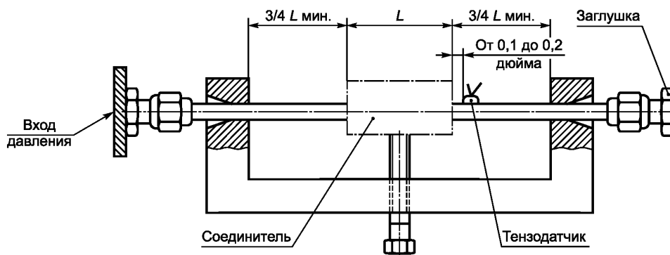
а) Испытательная установка для прямого соединителя
