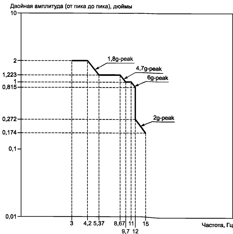
Рисунок 10 — Кривая 1AF
