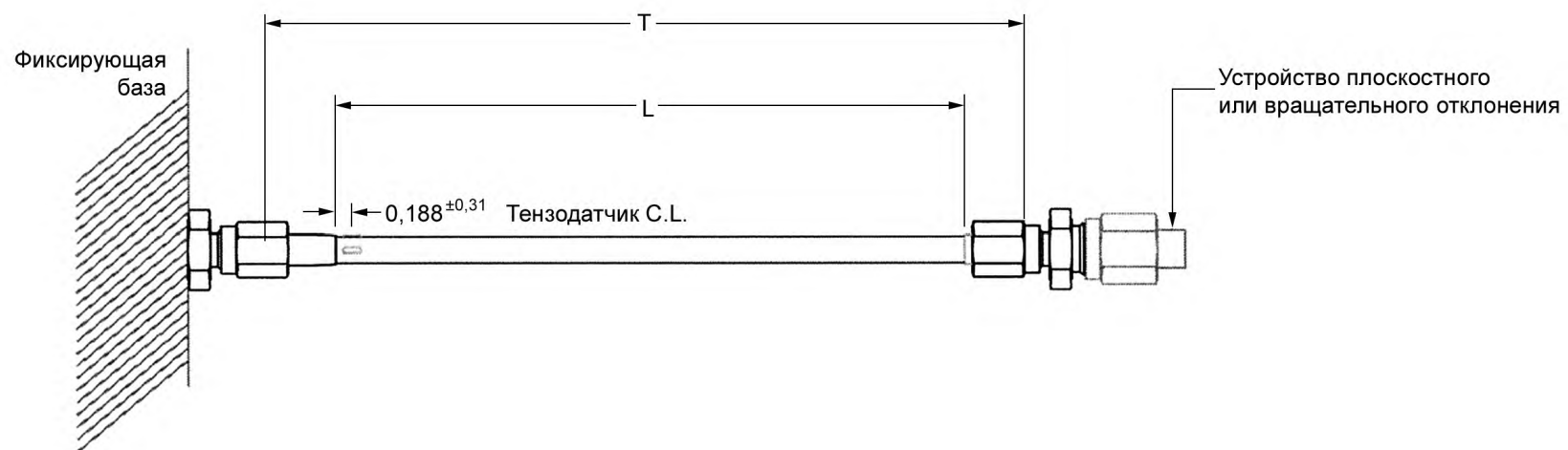
Рисунок 2 — Образец при испытаниях вращением или изгибом в плоскости
