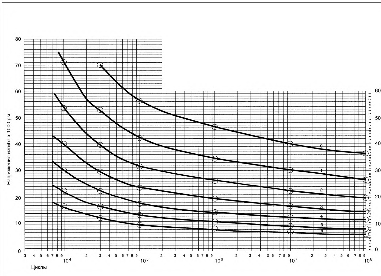
Рисунок 1 — S/N кривая испытания на усталостное разрушение при изгибе
