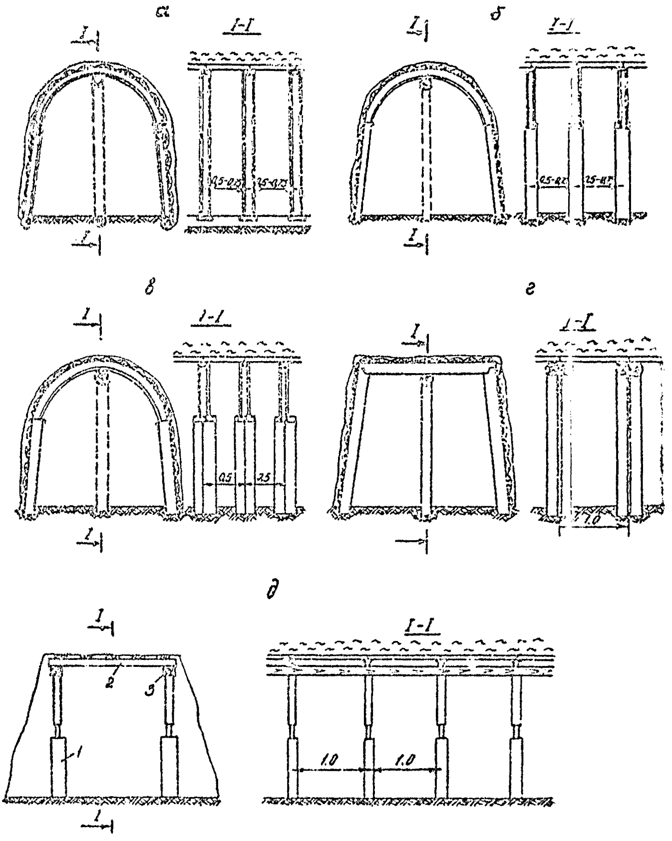
Рис. 1. 6. - варианты конструкции
