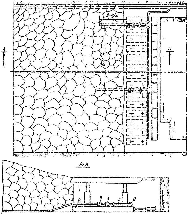
Рис. 18. Схема расположения передвижного пылесосового а в лава с комплексом КМ-873
