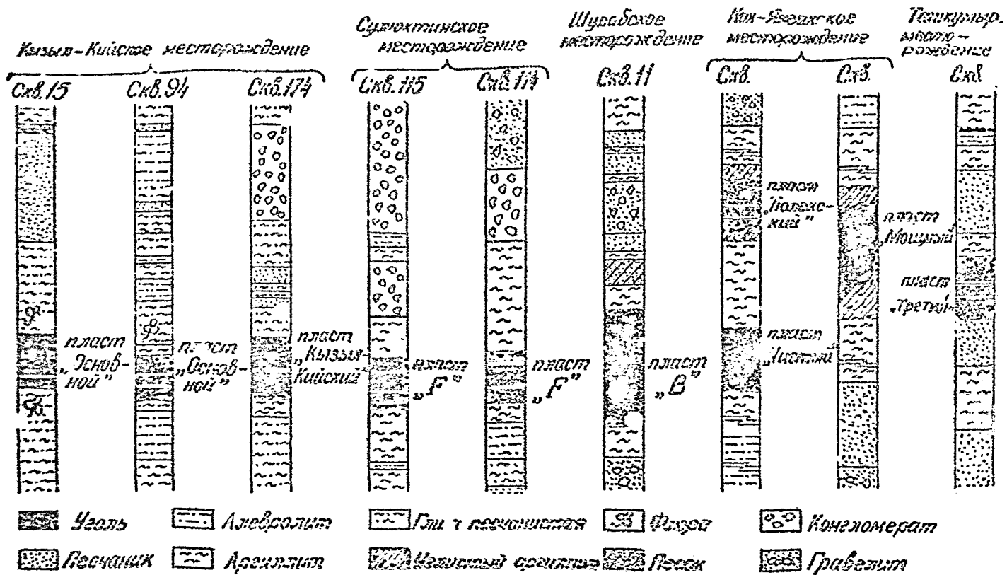
Рис. 1. Литологические колонки пород угленосной толщи месторождений Южно-Ферганского района
