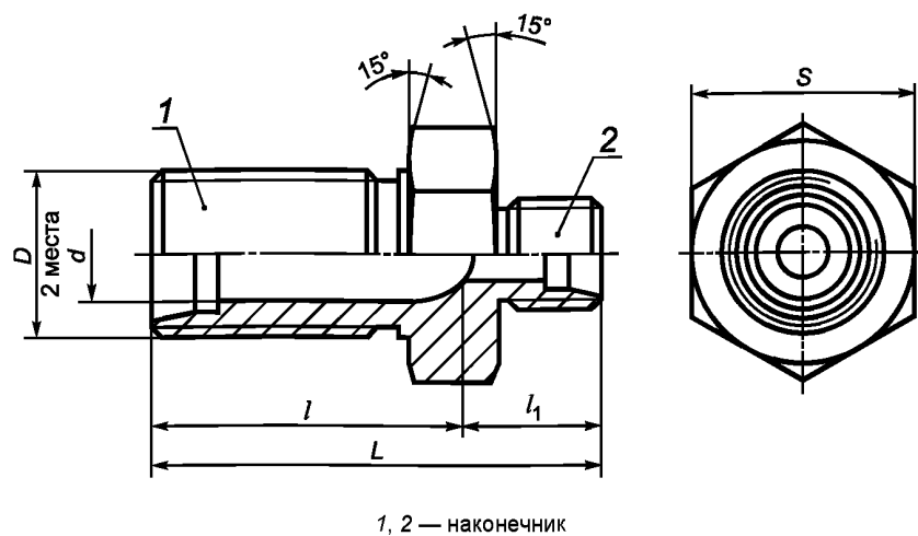
Рисунок 1 — Проходник (переходник)
