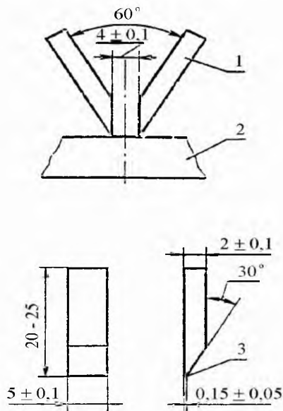
1 – электрод; 2 – образец; 3 – закругленный край
