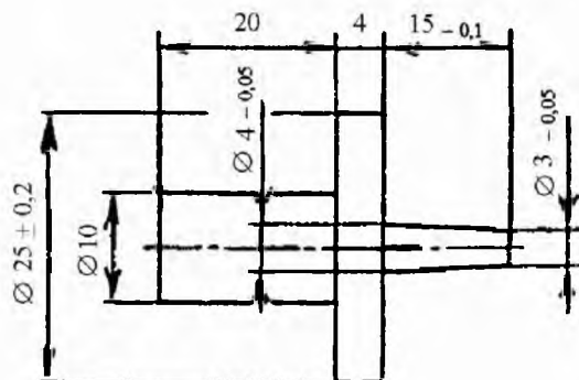
Рисунок 2 – Испытательный щуп
