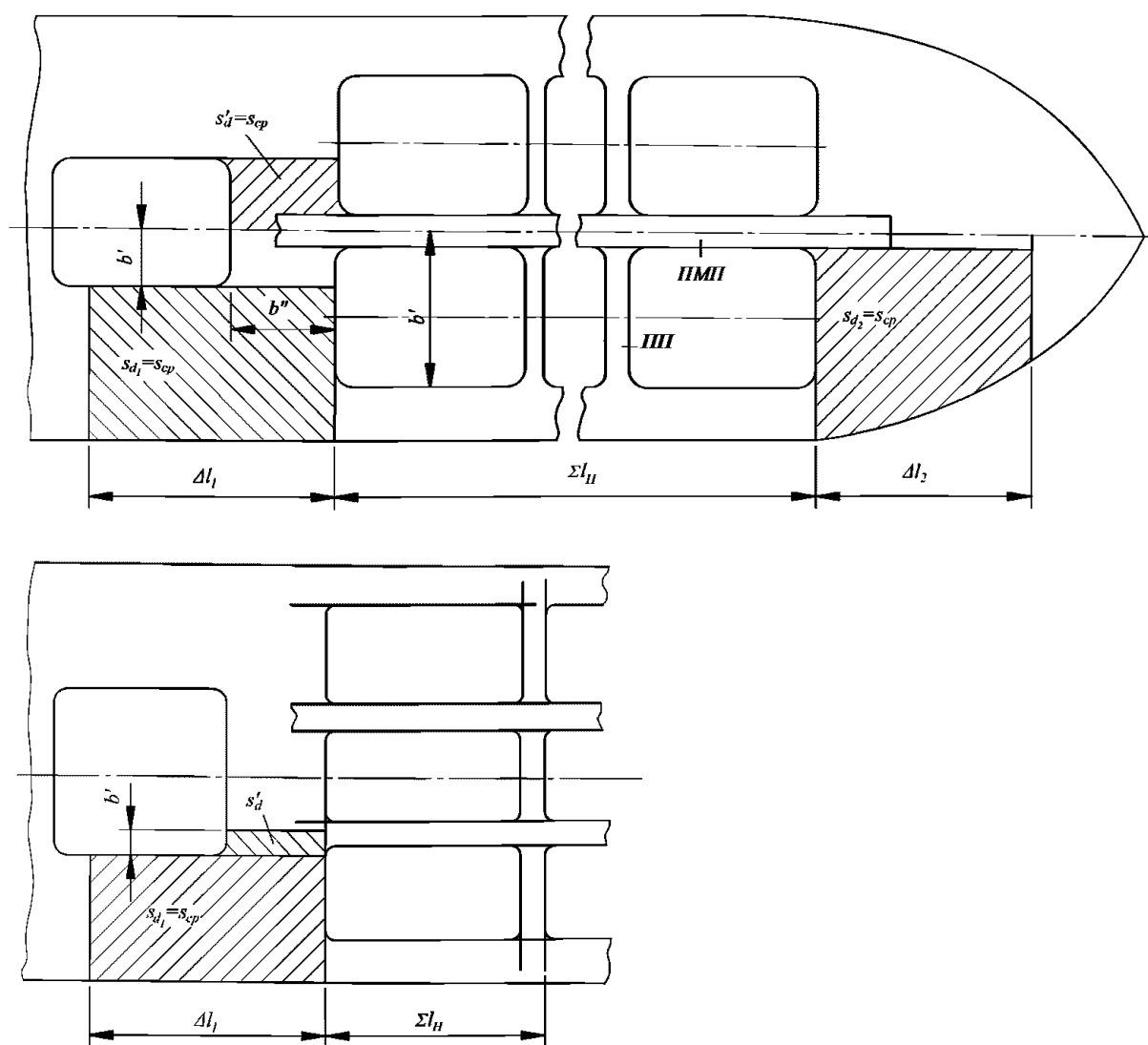
Рис. 1.4.8.2 Учет продольных межпалубных перемычек при определении момента сопротивления поперечного сечения корпуса
