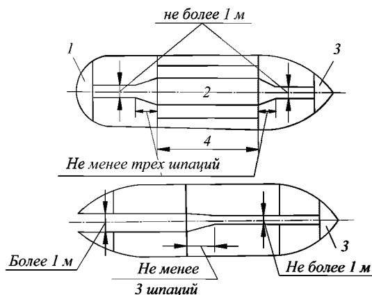
Рис. 3.6.2.4.1: 1 — ахтерпик; 2 — килевая балка; 3 — форпик; 4 — грунтовой трюм
