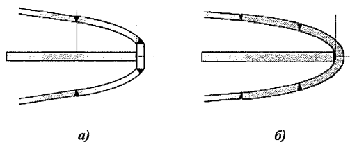
Рис. 3.10.2.6.2-1 Конструкция форштевня: а) комбинированный; б) листовой
