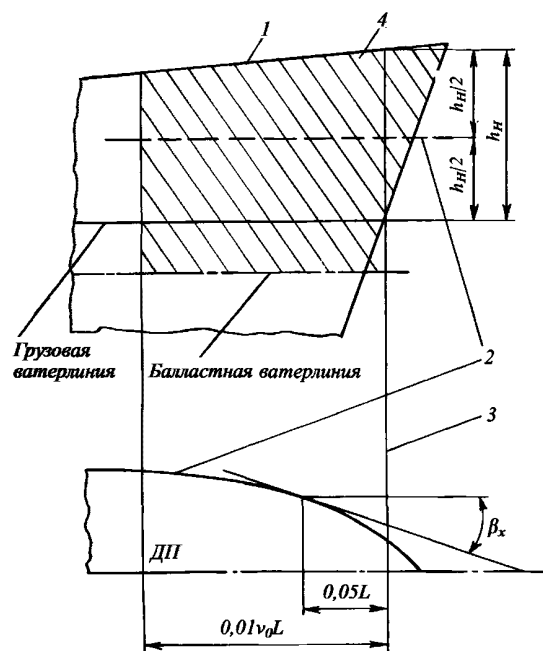
Рис. 2.8.1.2-2 Схема определения угла \beta_x и области действия ударного давления волн (заптрихована): 1 — верхняя открытая палуба; 2 — ватерлиния для определения угла \beta_x ; 3 — носовой перпендикуляр; 4 — область ударных давлений; h_n — вертикальное расстояние между ГВЛ и верхней открытой палубой на носовом перпендикуляре
