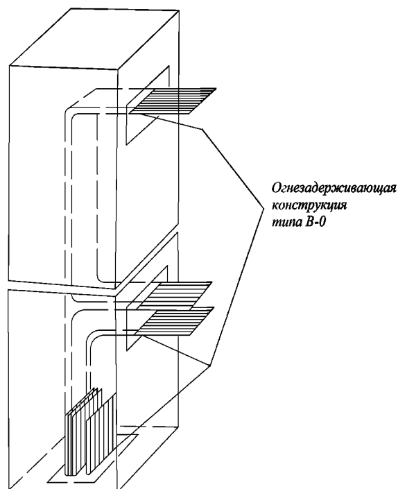
Рис. 16.8.4.3.1 Защита полностью закрытой кабельной трассы типа В-0
