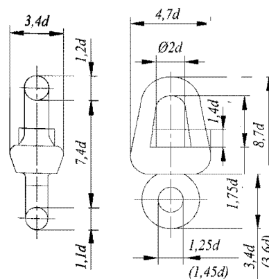
Рис. 7.1.3-7 Вертилог
