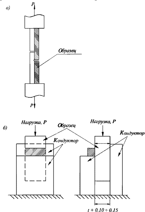
Рис. 5.3.2.3.4.3.2-2 Схемы испытания на срез (а или б)
