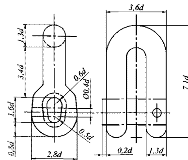
Рис. 7.1.3-5 Соединительная скоба
