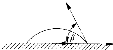
Рис. 2.5.7.1 Смачиваемость твердого тела жидкостью: β – краевой угол смачивания
