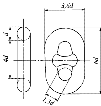
Рис. 7.1.3-1 Обычное звено
